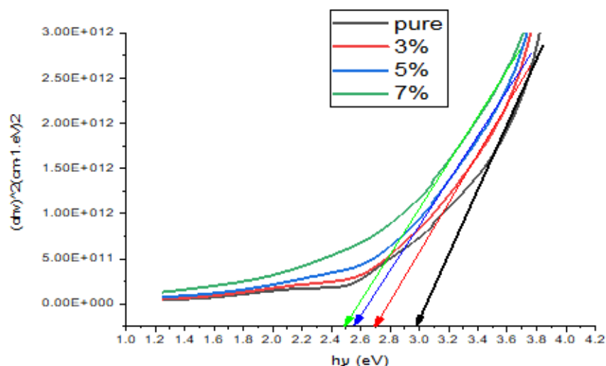
الشكل (7) : منحي فجوة الطاقة لأغشية (ZnSe) النقية والمشوبة عند (500) نبضة .
