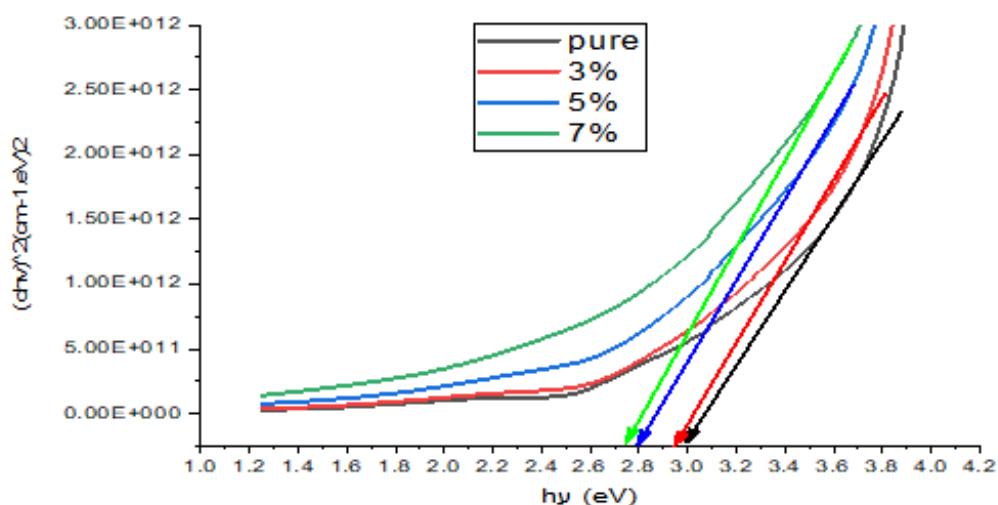
الشكل (6) : منحي فجوة الطاقة لأغشية (ZnSe) النقية والمشوبة عند (100) نبضة .
