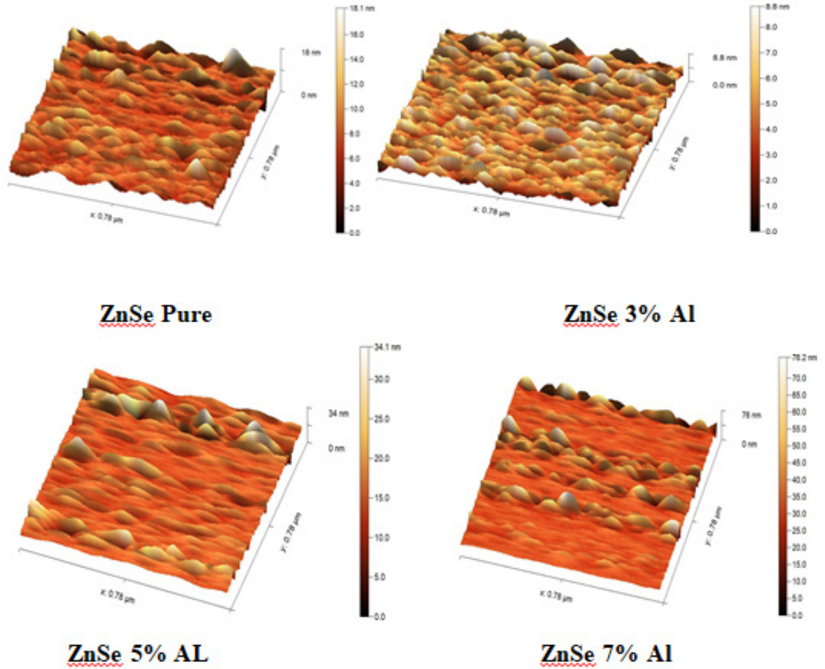
الشكل (4) : صور (AFM) للأغشية (ZnSe) النقية والمشوبة المحضرة عند (100) نبضة .
