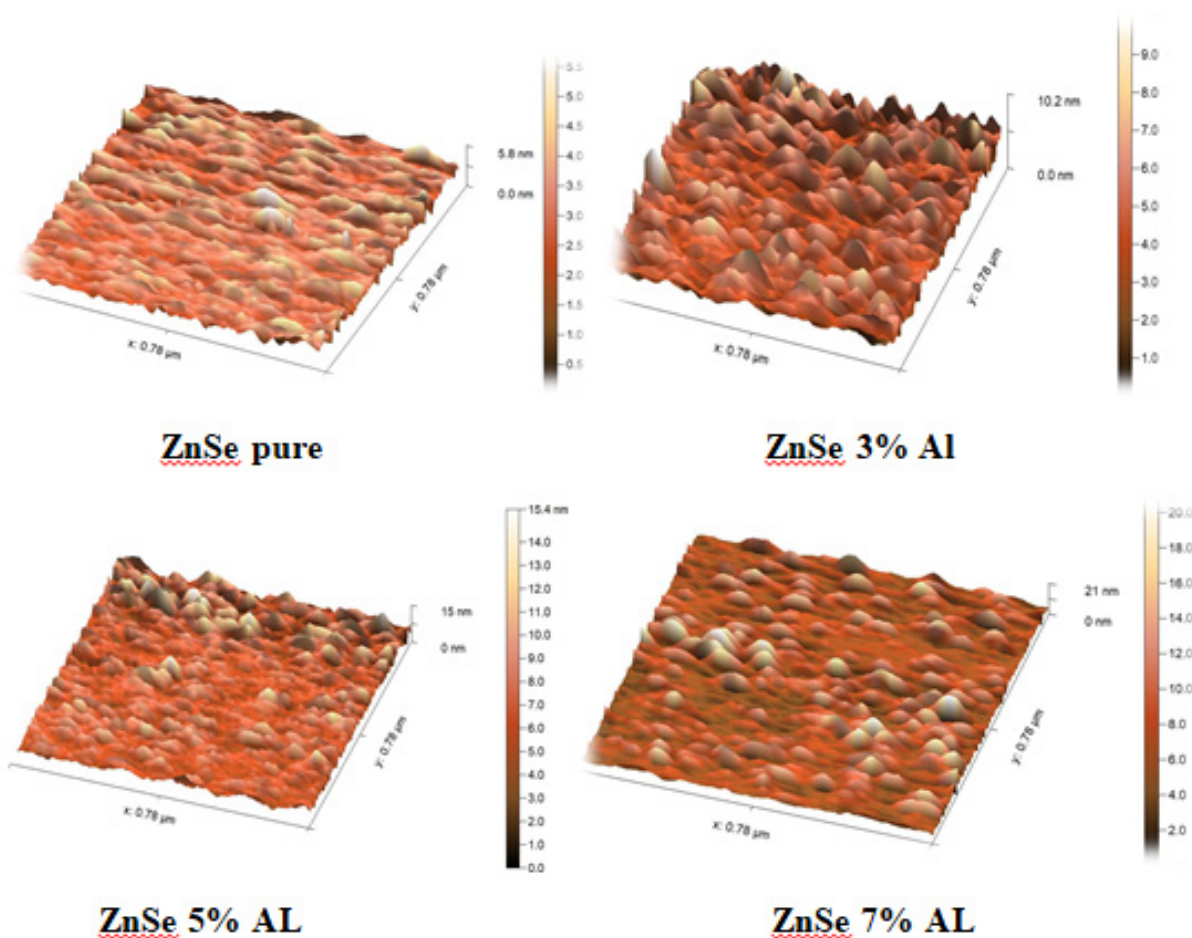
الشكل (5): صور (AFM) لأغشية (ZnSe) النقية والمشوبة عند (500) نبضة .
