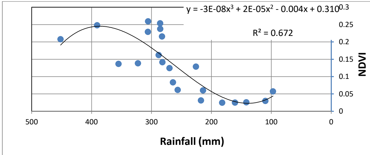
الشكل (٨) يبين النموذج الرياضي المقترح للعلاقة بين قيم NDVI وكمية الامطار الساقطة
