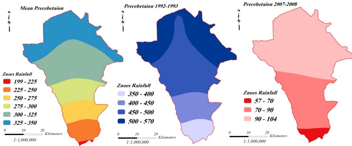
الشكل (٦) يوضح نموذجين لسنة مطيرة (١٩٩٢-١٩٩٣) وسنة جافة (٢٠٠٧-٢٠٠٨)
