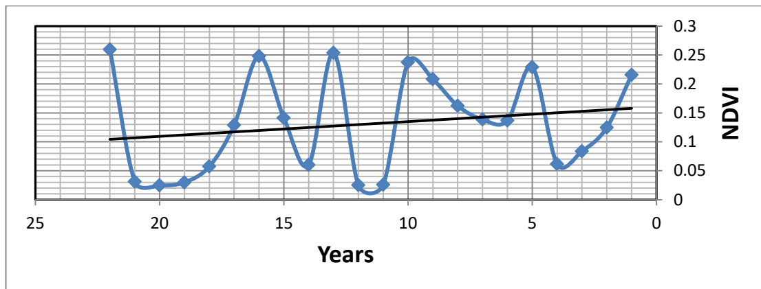
الشكل (٥) الاتجاه العام لقيم NDVI لمنطقة الدراسة للفترة من ١٩٨٥ - ٢٠١٤
