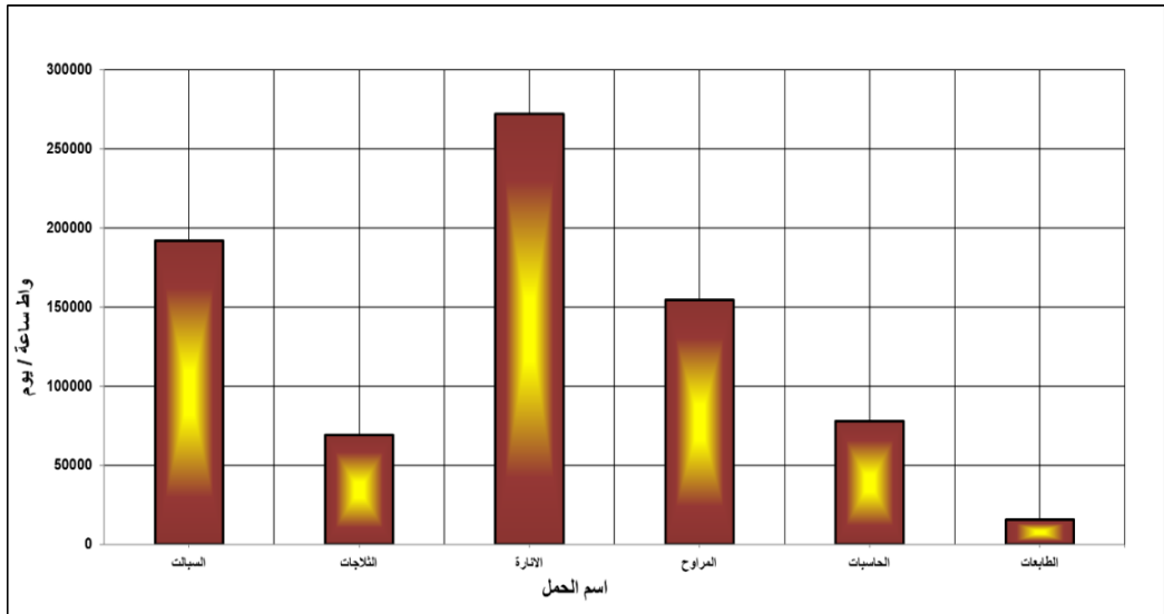
شكل (٣) قدرة الاحمال وساعات التشغيل في مجمع عرعر.
