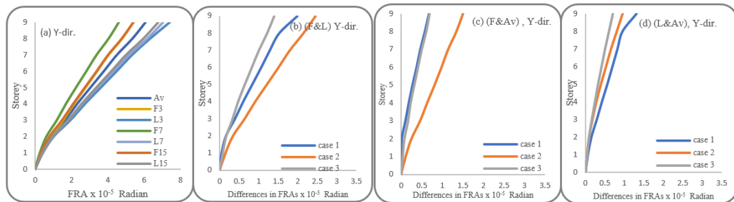
Figure12. FRAs and DFs of Cases 1-3 in, the Y-direction (a) FRAs (b) F&L (C) F&Av (d) L&Av
