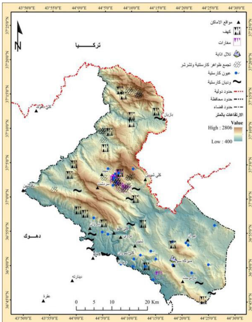
الخريطة ( 2 ) الكهوف الكارستية في منطقة الدراسة
