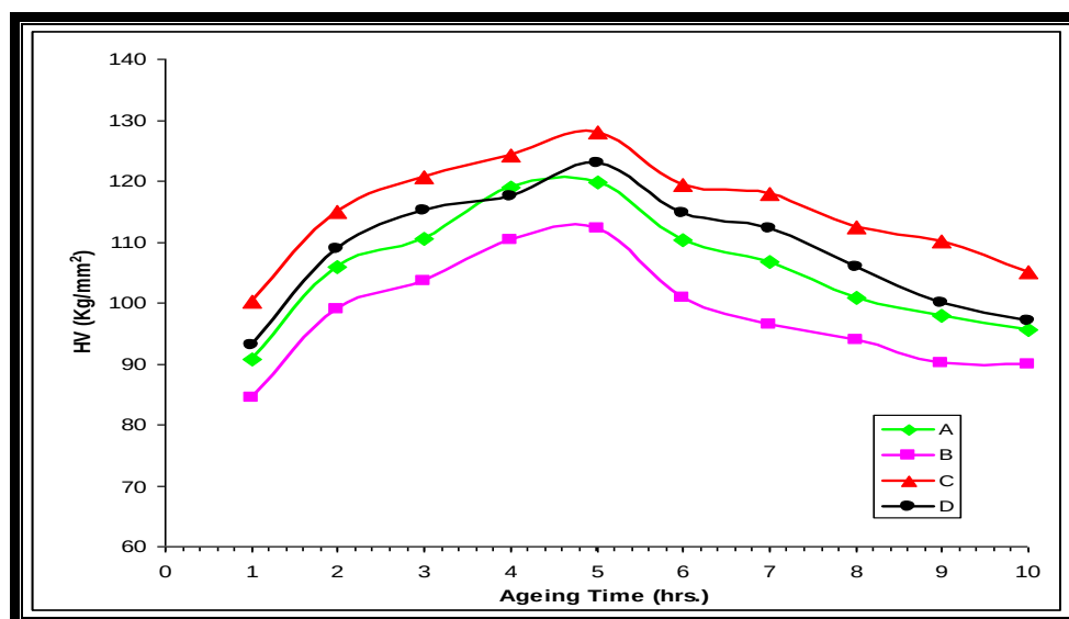
الشكل ( 3 ) العلاقة بين الصلادة الدقيقة و زمن التعتيق الاصطناعي للسبائك (A,B,C,D) عند درجة حرارة تعتيق (175°C) .
