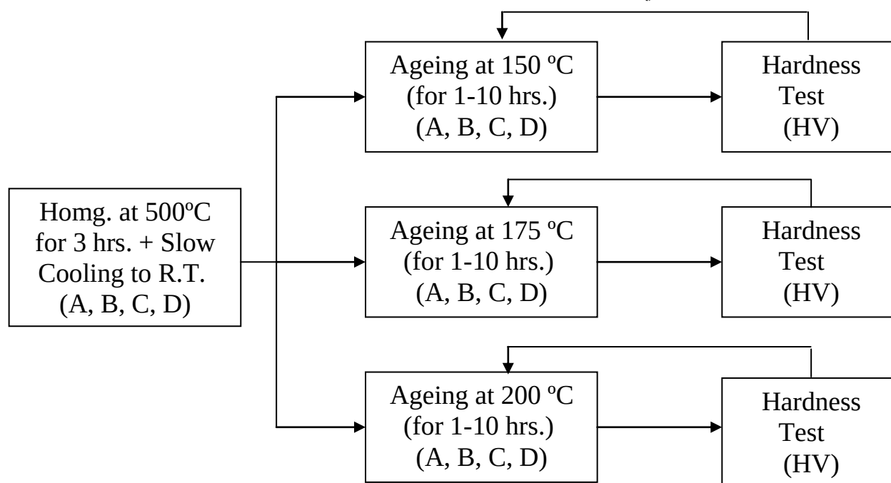
شكل (1) مخطط عملية التعتيق الاصطناعي مع قياس الصلادة .
