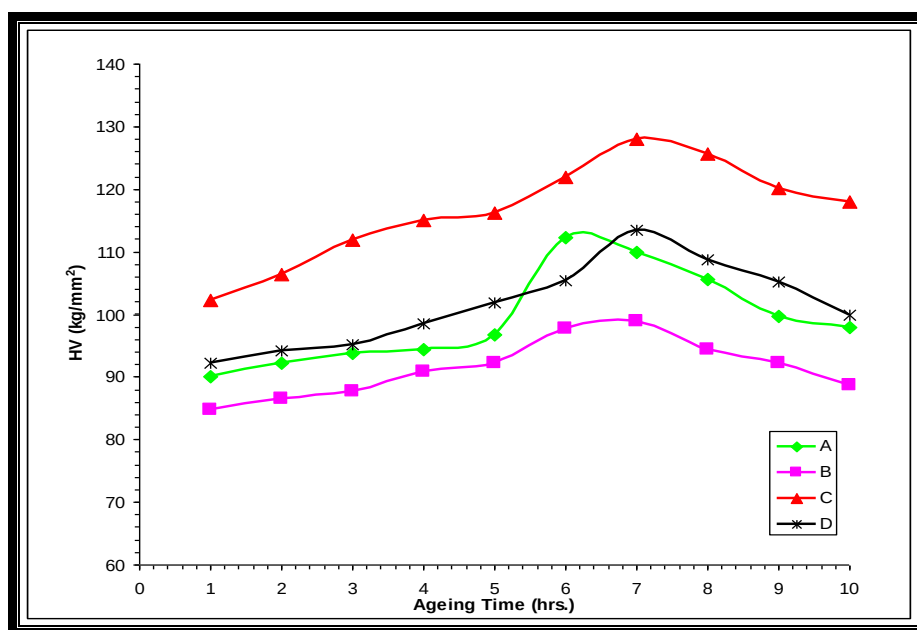
الشكل (2) العلاقة بين الصلادة الدقيقة و زمن التعتيق الاصطناعي للسبائك (A,B,C,D) عند درجة حرارة تعتيق (150°C).
