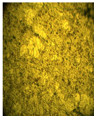
الشكل (9) البنية المجهرية للسبيكة (C) بعد التعتيق بدرجة حرارة (175 °C) .
