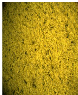
الشكل (8) البنية المجهرية للسبيكة (A) بعد التعتيق بدرجة حرارة (150 °C) .
