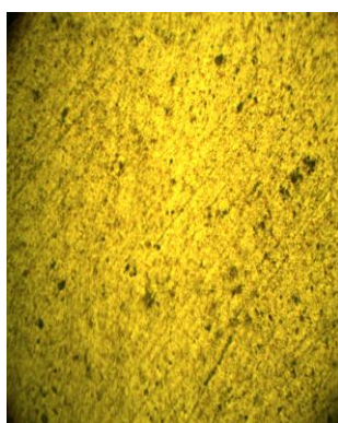
الشكل (10) البنية المجهرية للسبيكة (D) بعد التعتيق بدرجة حرارة (200 °C) .
