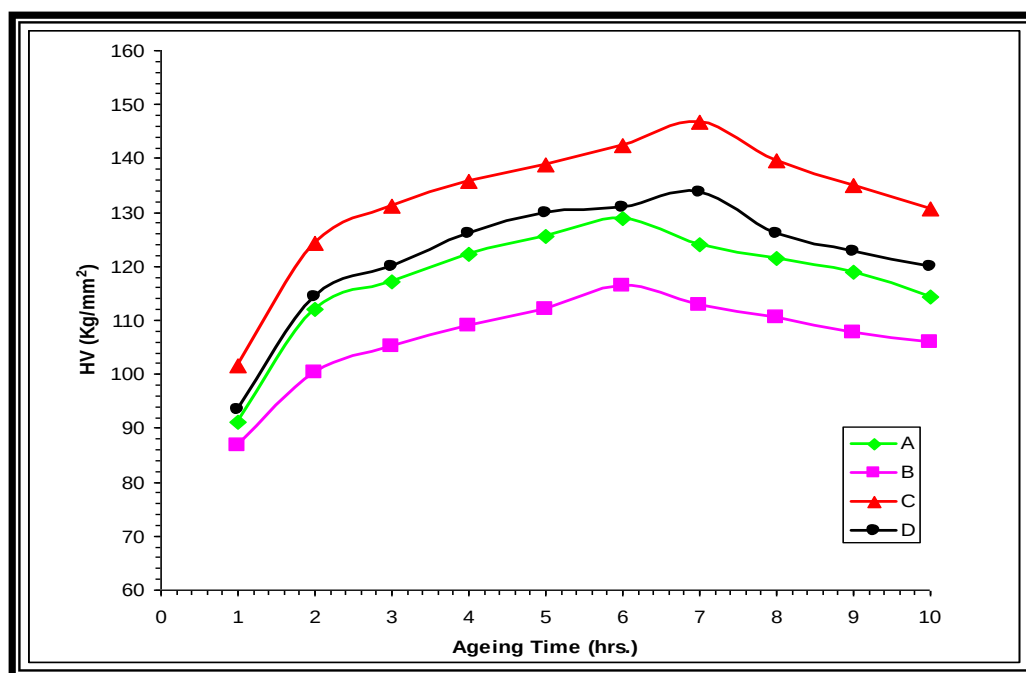
الشكل ( 3 ) العلاقة بين الصلادة الدقيقة و زمن التعتيق الاصطناعي للسبائك (A,B,C,D) عند درجة حرارة تعتيق (175°C) .
