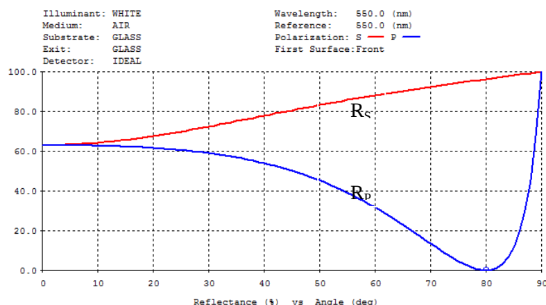
شكل (9) الانعكاسية دالة لزاوية السقوط للضوء لطلاء مضاد للانعكاس لنمط الاستقطاب P- مكون من ثلاث طبقات مرسبة على الزجاج عند زاوية السقوط ( \theta_0=80^\circ ) للتصميم النهائي (الامثل)
