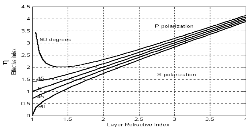
شكل (2) معامل الانكسار الفعال \eta دالة للتغير في قيم معامل الانكسار الحقيقي للمواد n ولزوايا السقوط ( 0^\circ, 45^\circ, 90^\circ )
