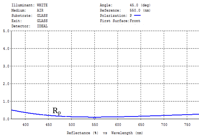
شكل (3) الانعكاسية دالة للطول الموجي لنمط الاستقطاب-P لطلاء مضاد للانعكاس ذو طبقة مفردة مرسبة على الزجاج عند زاوية السقوط ( \theta_o = 45^\circ ) للتصميم (n_L = 1.38) \text{ Air} | L | \text{ glass}
