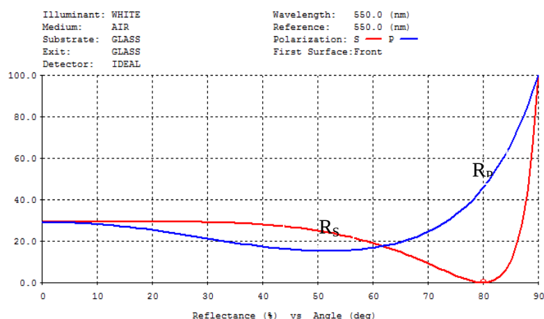
شكل (10) الانعكاسية دالة لزوايا السقوط للضوء لطلاء مضاد للانعكاس لنمط الاستقطاب S- مكون من ثلاث طبقات مرسبة على الزجاج عند زاوية السقوط ( \theta_0 = 80^\circ ) للتصميم النهائي (الامتثل) (Air | 0.925L1.174H1.416L | glass)
