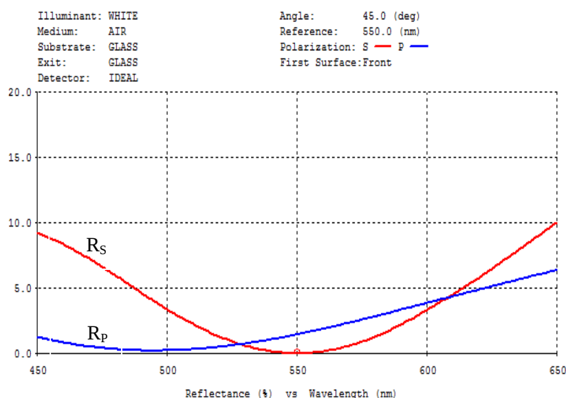
شكل (5) الانعكاسية دالة للطول الموجي لنمطي الاستقطاب لطلاء مضاد للانعكاس مكون من طبقتين مرسبة على الزجاج عند زاوية السقوط ( \theta_0=45^\circ ) للتصميم Air [1.730H0.820L]glass ( n_L=1.6 ), ( n_H=2.45 )
