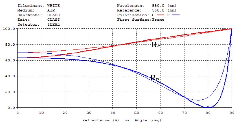
شكل (11) مقارنة الانعكاسية دالة لزوايا السقوط للضوء لنمط الاستقطاب P- لطلاء مضاد للانعكاس مكون من ثلاث طبقات مرسبة على الزجاج عند زاوية السقوط ( \theta_0 = 80^\circ ) للتصميم الابتدائي (المنحني الفاتح)
