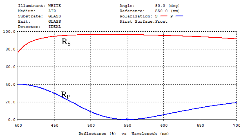
شكل (7) الانعكاسية دالة للطول الموجي لطلاء مضاد للانعكاس لنمط الاستقطاب P- مكون من ثلاث طبقات عند زاوية السقوط ( \theta_0=80^\circ ) للتصميم (Air | 1.054H1.105L1.266H | glass) ( n_L=1.48 ), ( n_H=2.4 )
