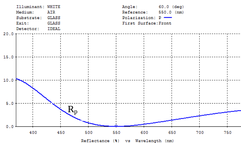
شكل (4) الانعكاسية دالة للطول الموجي لنمط الاستقطاب-P لطلاء مضاد للانعكاس ذو طبقة مفردة مرسبة على الزجاج عند زاوية السقوط ( \theta_o = 60^\circ ) للتصميم \text{Air} | H | \text{glass}
