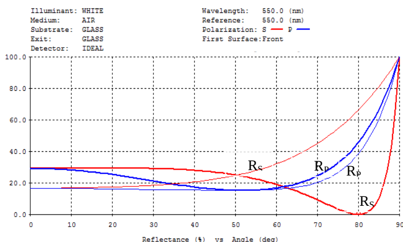
شكل (12) مقارنة الانعكاسية دالة للطول الموجي لنمط الاستقطاب S- لطلاء مضاد للانعكاس مكون من ثلاث طبقات مرسبة على الزجاج عند زاوية السقوط ( \theta_0 = 80^\circ ) للتصميم الابتدائي (المنحني الفاتح) والنهائي (الامتثل) (المنحني الغامق)
