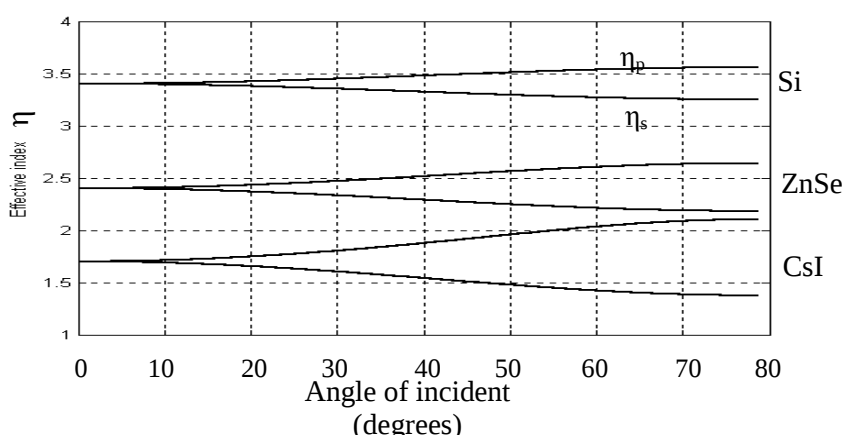
شكل (1) السماحية البصرية لنمطي الاستقطاب العمودي والموازي ولزوايا السقوط من الهواء إلى مواد ذات معاملات انكسار مختلفة
