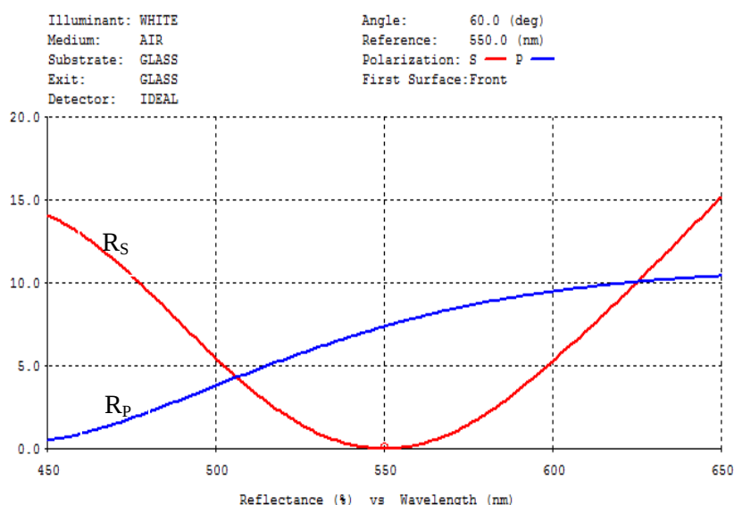
شكل (6) الانعكاسية دالة للطول الموجي لنمطي الاستقطاب لطلاء مضاد للانعكاس مكون من طبقتين مرسبة على الزجاج عند زاوية السقوط ( \theta_0=60^\circ ) للتصميم Air [1.640H0.972L]glass ( n_L=1.48 ), ( n_H=2.4 )
