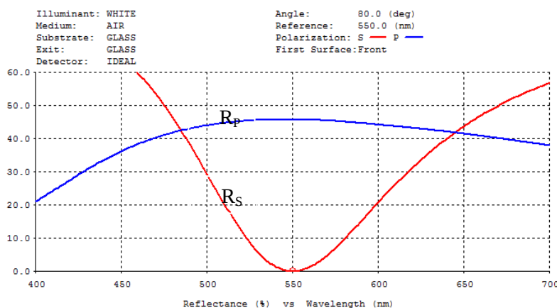
شكل (8) الانعكاسية دالة للطول الموجي لطلاء مضاد للانعكاس لنمط الاستقطاب S- مكون من ثلاث طبقات عند زاوية السقوط ( \theta_0=80^\circ ) للتصميم (Air | 0.925L1.174H1.416L | glass) ( n_L=1.48 ), ( n_H=2.4 )
