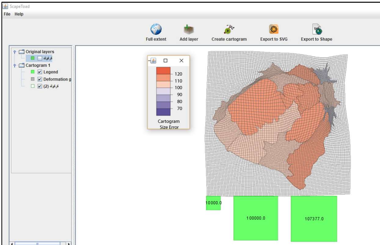
شكل (١) فكرة عمل أداة الكارتوكرام المتصل
