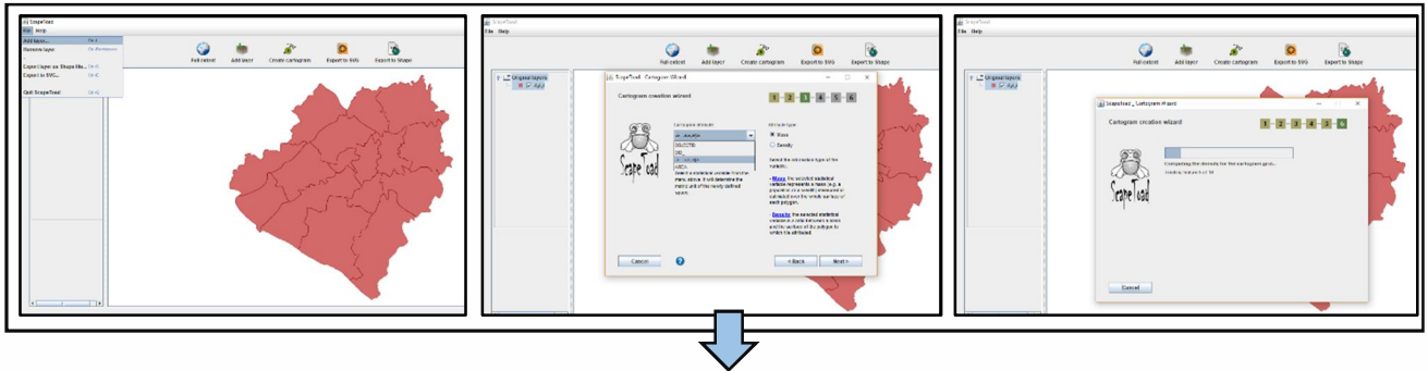
شكل (٢) خطوات العمل لاشتقاق الكارتوكرام المتصل
