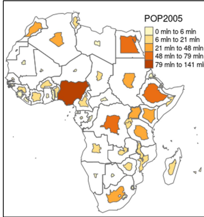
شكل (٣) فكرة عمل الكارتوكرام المنفصل
