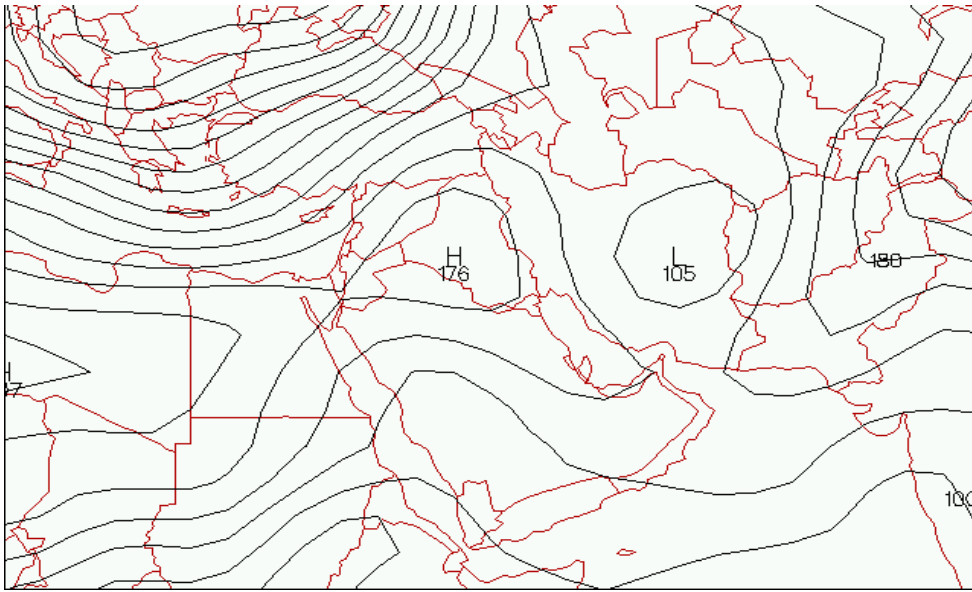
خريطة (3) سيطرة المرتفع شبه المداري على العراق بتاريخ 1999\12\27 الرصدة (12:00) GMT
