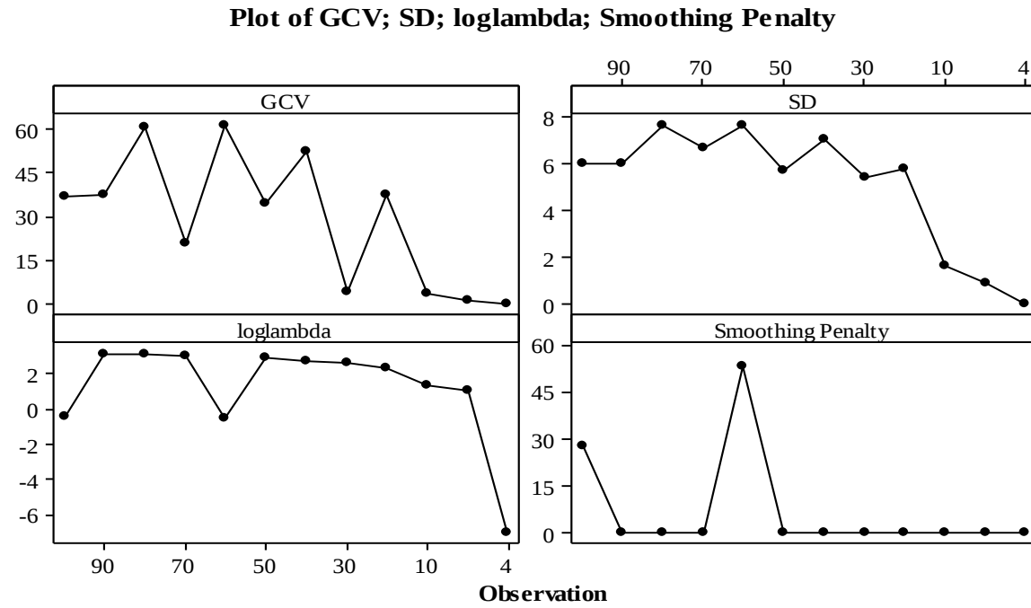
الشكل (1): يوضح الرسوم البيانية لإحصاءات التقديرات النهائية الواردة في الجدول (1) للانموذج الخطي في ظل وجود المشاهدات الشاردة، ولحجوم عينات مختلفة
