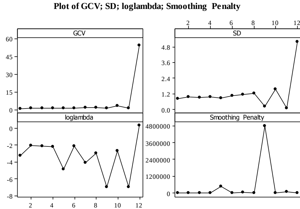
الشكل (5): يوضح الرسوم البيانية لإحصاءات التقديرات النهائية الواردة في الجدول (3) للنموذج اللاخطي في ظل وجود المشاهدات الشاردة، ولحجوم عينات مختلفة
