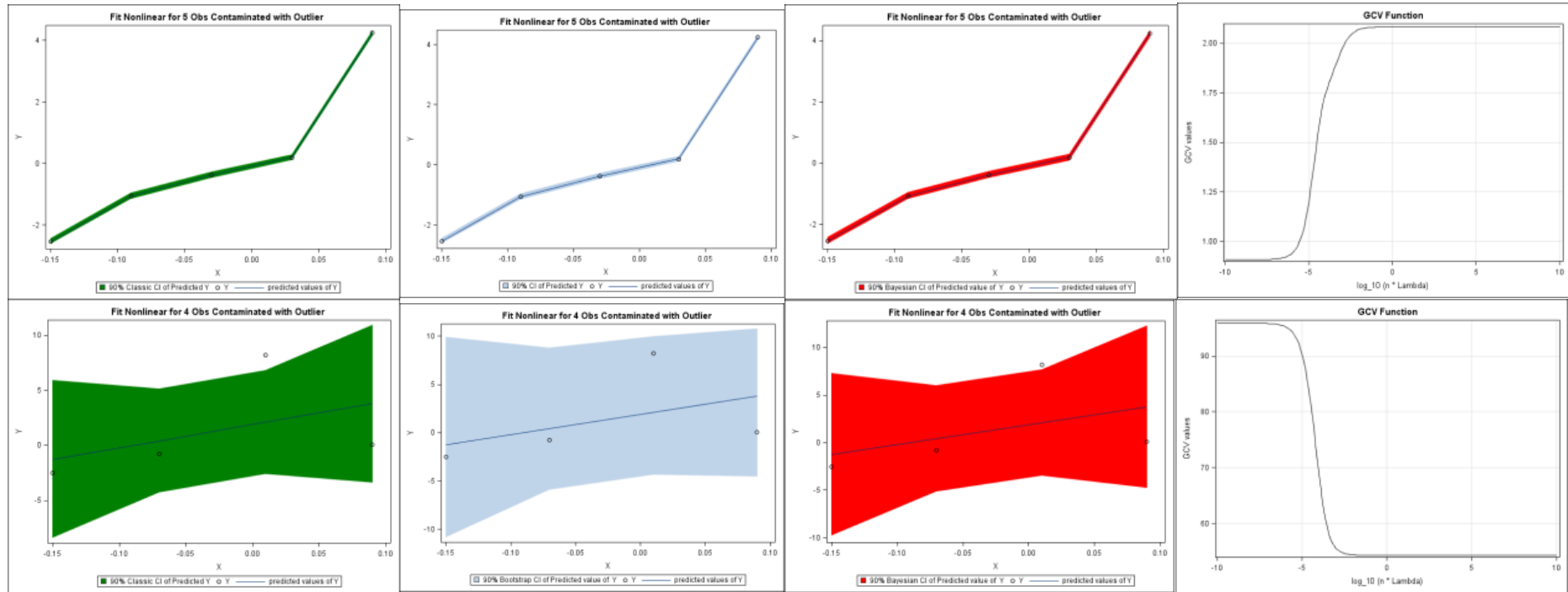
الشكل (6): يوضح الرسوم البيانية لكل من حدود الثقة بوتستراب والبيزية والكلاسيكية، فضلاً عن الرسم البياني لدالة الصلاحية التقاطع المعممة للنموذج اللاخطي في ظل وجود المشاهدات الشاردة ولحجوم عينات مختلفة.
