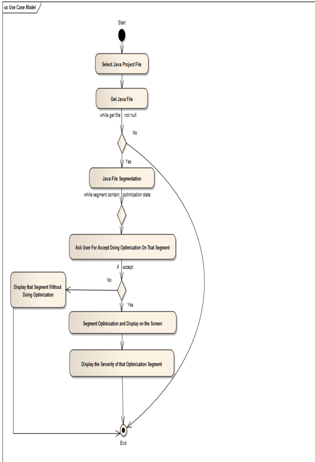
الشكل (5): مخطط الفعالية للأداة المقترحة JCOT
