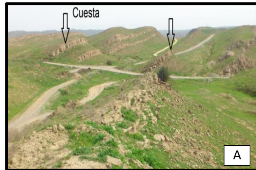
لوحة (2) (A) ظاهرة Cuesta من مقطع سلسلة كركوك (الديس)
