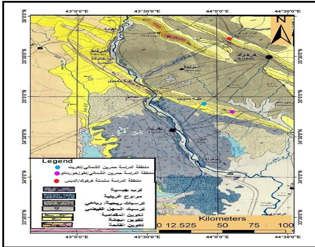
شكل (1) خارطة جيولوجية توضح موقع مقاطع الدراسة الثالث
