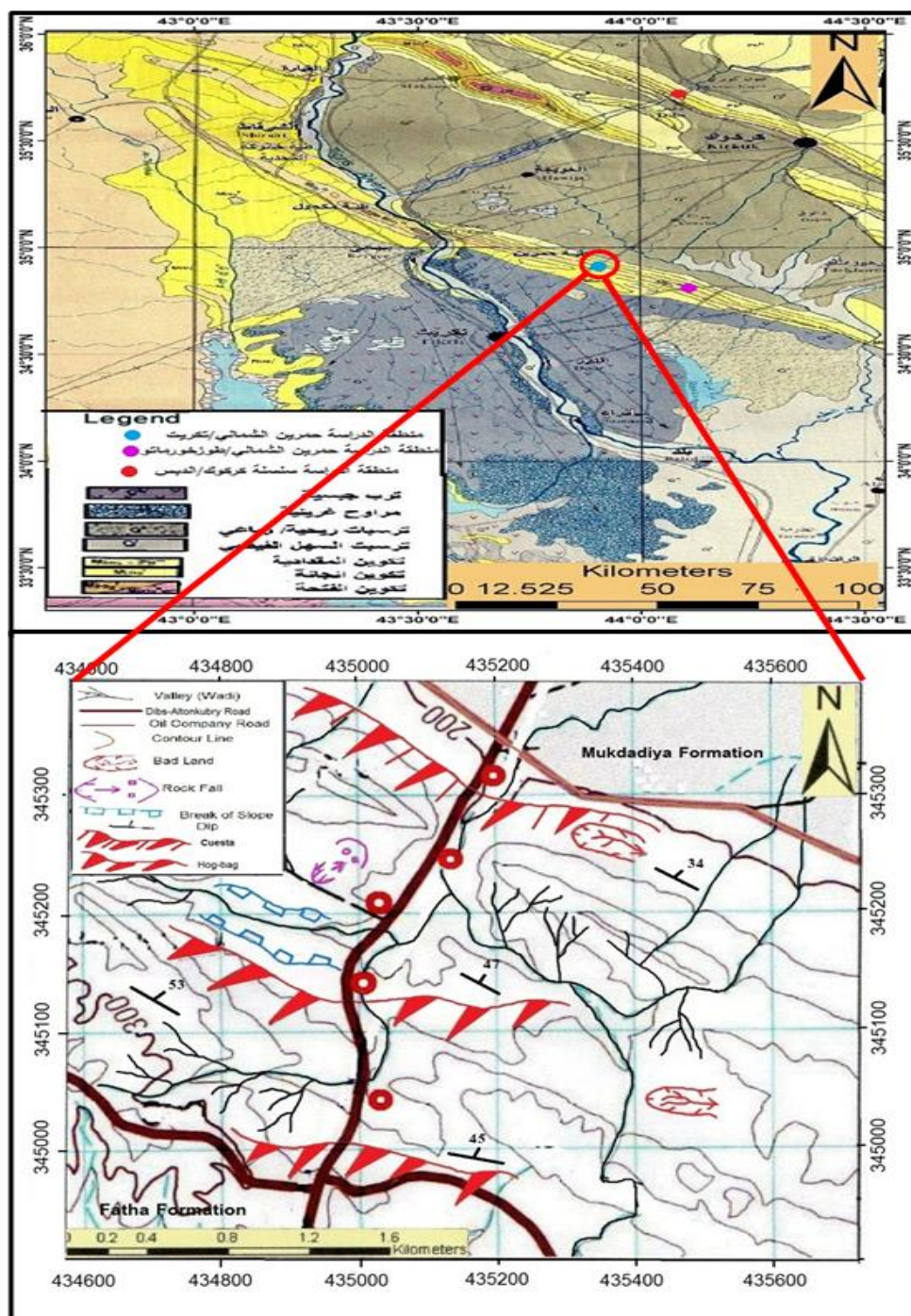
شكل (4). الخطة الجيومورفولوجية لمنطقة الدراسة حوض التيمالي / تكريت
