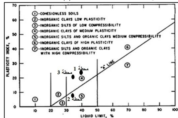
شكل (7) مخطط اللدونة موضحا عليه محطات منطقة الدراسة
