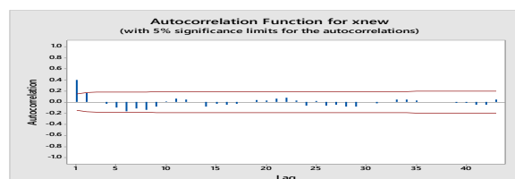
الشكل (3) رسم ACF & PACF لسلسلة الإدخال بعد الاستقرارية
