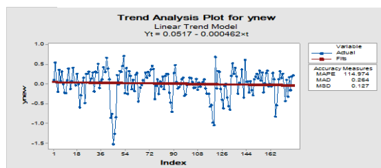
سلسلة المخرجات بعد استقراريتها
