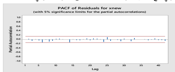
الشكل (4) رسم ACF & PACF لبواقي افضل نموذج ARIMA(1,1,0)
