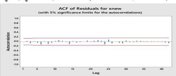
الشكل (4) رسم ACF & PACF لبواقي افضل نموذج ARIMA(1,1,0)
