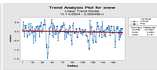
سلسلة المدخلات بعد استقراريتها
