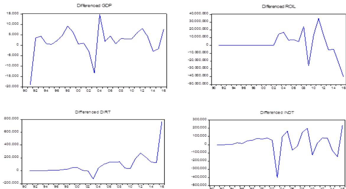
شكل (٢) الاستقرار عند الفرق الأول
