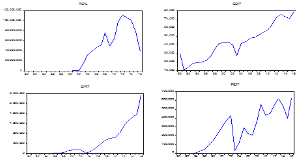
شكل (١) الاستقرار عند المستوى
