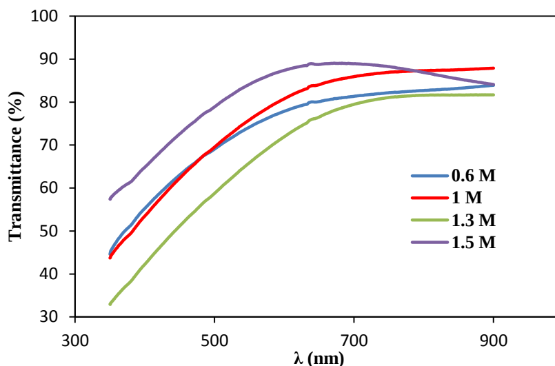
شكل 3: طيف النفاذية لغشاء (\text{Cu}_2\text{S}) الرقيق المحضر بتغيير قيم التراكيز المولارية (M) لمادة
