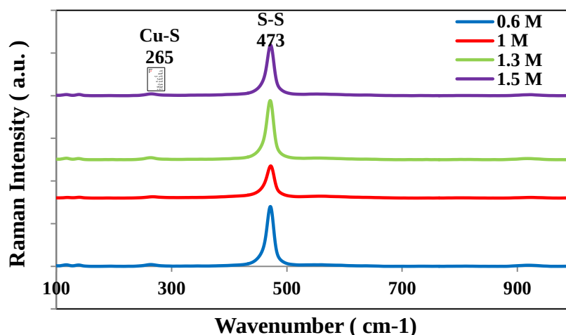
الشكل 12: مطياف رامان لأغشية (Cu 2 S) الرقيقة ذات البنية النانوية والمحضرة بتغيير في التركيز المولاري (M) لمادة
