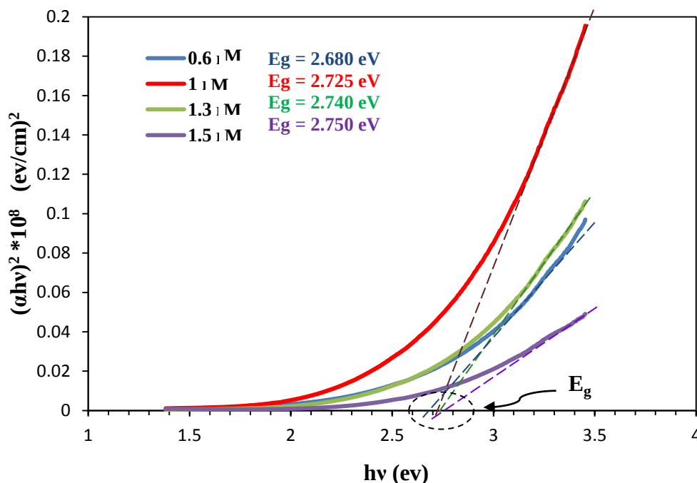
شكل 6: قيمة فجوة الطاقة المباشرة E_g لغطاء (\text{Cu}_2\text{S}) الرقيق المحضر بتغيير قيم التركيز المولارية ( M ) لمادة
