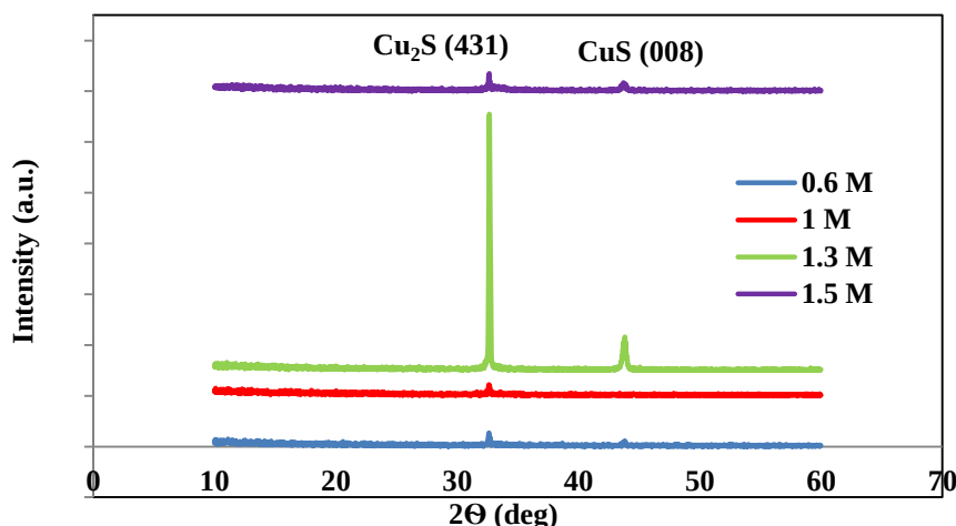
الشكل 2: طيف شدة حيود الأشعة السينية لأغشية (Cu 2 S) الرقيقة بتغيير التركيز المولاري (M) لمادة
