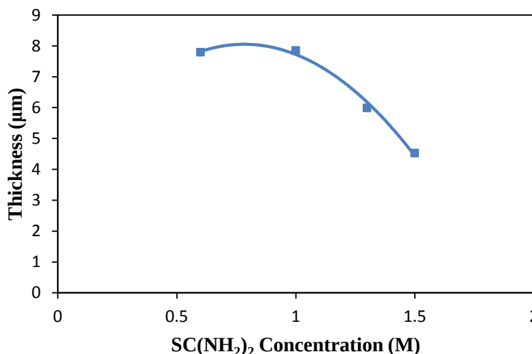
شكل 4: تغير سمك الغشاء (\text{Cu}_2\text{S}) الرقيق المحضر بتغيير قيم التراكيز المولارية (M) لمادة الثايويوريا [\text{CS}(\text{NH}_2)_2]
