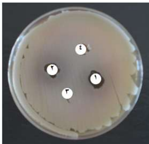
E. coli
