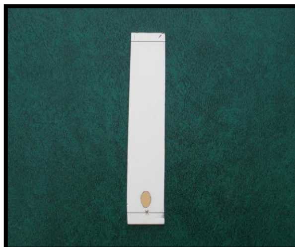
صورة (١): كروماتوغرافيا الطبقة الرقيقة للفايسين
