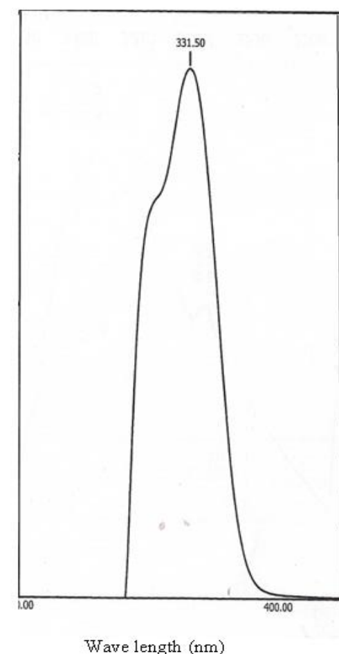
شكل (٤) طيف المنطقة فوق البنفسجية لمركب الفايسين القياسي في مذيب الايثانول (Dutta وجماعته ، ١٩٨١)
