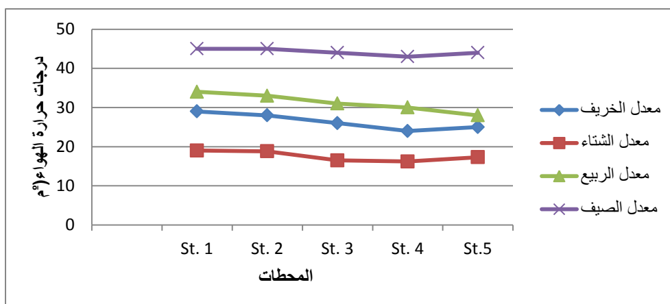
شكل (2) التغيرات الفصلية لدرجة حرارة الهواء (°C) في محطات الدراسة.
