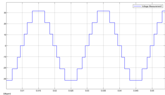
(d) Output voltage waveform using MATLAB Simulink
