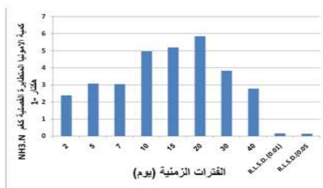
الشكل (٢) تأثير الفترات الزمنية المختلفة في كمية الامونيا المتطابرة الفعلية كغم NH 3 -N هكتار ١- بعد فترة 40 يوماً من اضافة السماد.
