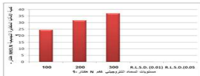
الشكل (٣) تأثير مستويات السماد النتروجيني في كمية الامونيا المتطايرة التجميعية كغم NH 3 -N هكتار-١ بعد فترة ٤٠ يوماً من اضافة السماد.
