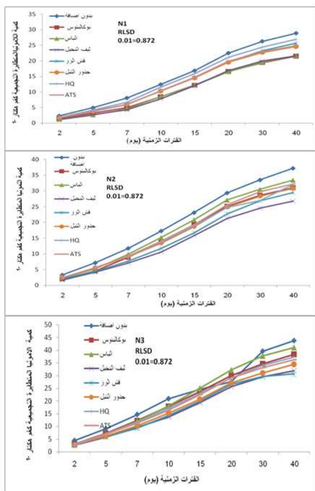
شكل (٥) تأثير التداخل لأنواع المستخلصات النباتية المائية والمركبات الكيميائية والفترات الزمنية في كمية الامونيا المتطايمة التجميعية للمستويات النتروجينية ١٠٠، ٢٠٠، ٣٠٠ كغم N هكتار -١
