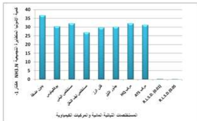
الشكل (١) تأثير أنواع المستخلصات النباتية المائية والمركبات الكيماوية في كمية الامونيا المتطايرة التجميعية كغم NH 3 -N هكتار -١ بعد ٤٠ يوما من اضافة السماد .
