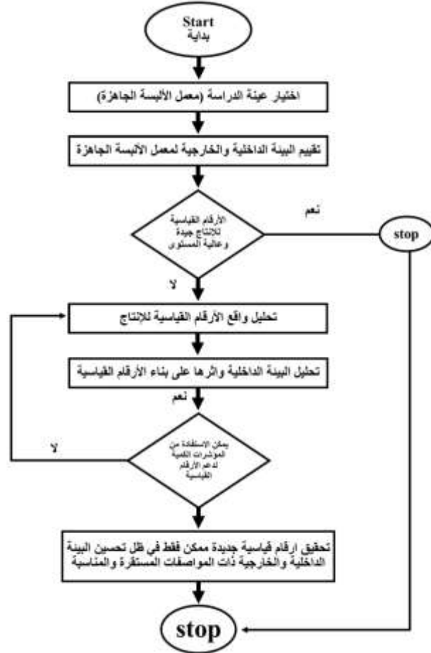
الشكل رقم (٦) المخطط الانسيابي الذي بموجبه تتم عملية تحقيق الأرقام القياسية
