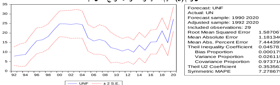
الشكل رقم (3) القيم الفعلية والمقدرة لأنموذج معدل البطالة
