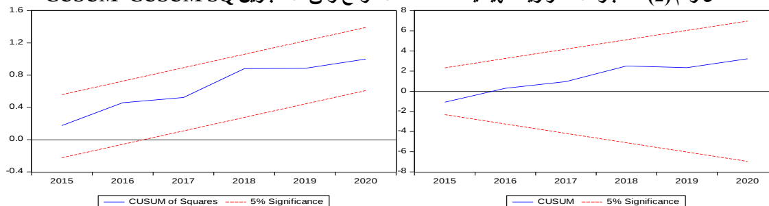
الشكل رقم (2) اختبار الاستقرار الهيكلية لمعاملات الانموذج وفق الاختبارين CUSUM-CUSUM SQ
