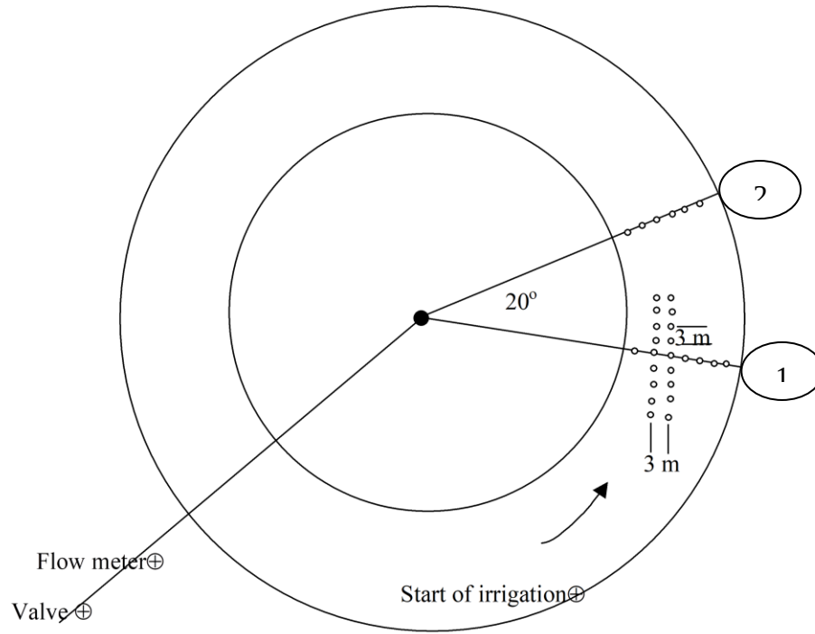
شكل-1: حدود التجربة الحقلية
