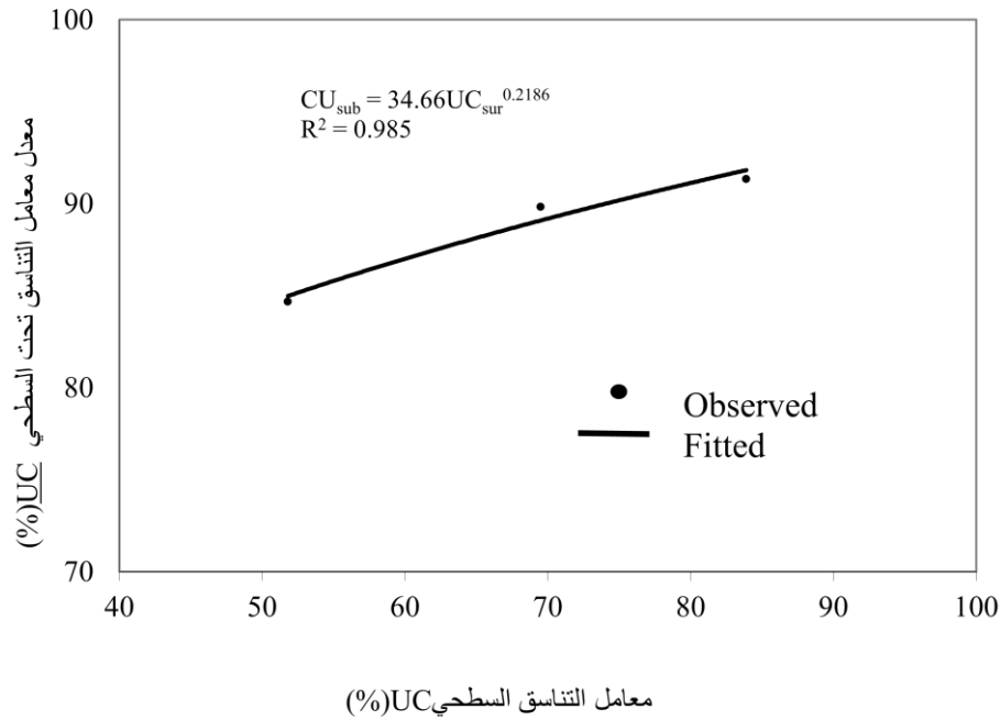
شكل-4: العلاقة بين معامل التناسق تحت السطحي والسطحي عمودياً على محور المنظومة
