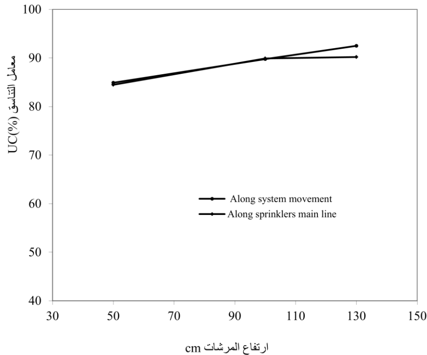
شكل-3: العلاقة بين معامل التناسق تحت سطحي وارتفاع المرشات
