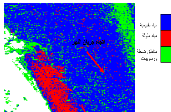
الشكل -9: التصنيف الموجه لمحطة مجاري السيلية للقمر
