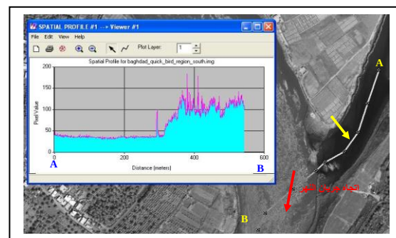
الشكل 8-: مقطع طولي لمنطقة التقاء نهر ديالى مع نهر دجلة لصورة القمر Quick bird
