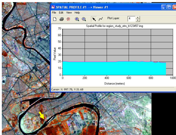
الشكل-3: مسار طولي profile بعد محطة كهرباء الدورة
