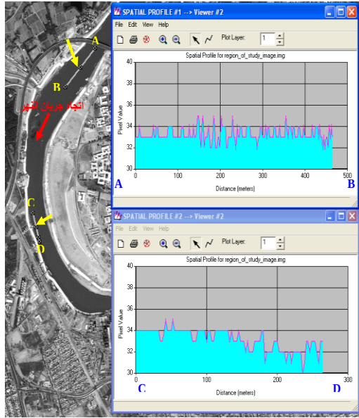
الشكل 5: مسار طولي للموقع 11 و 12 على صورة القمر الفرنسي Spot5
