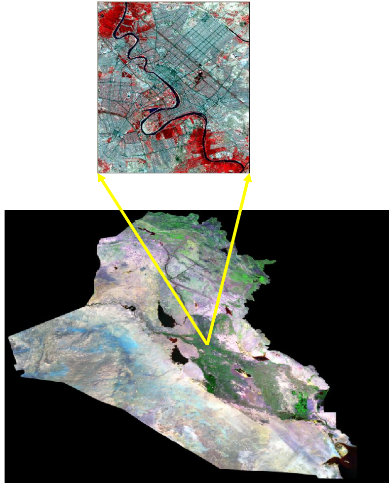
الشكل-1: صورة فضائية موضح عليها موقع منطقة الدراسة
