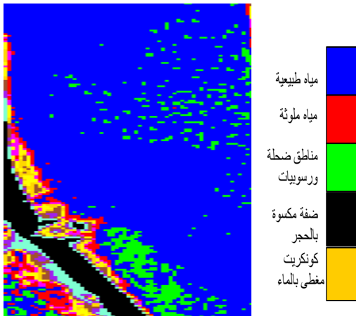
الشكل 6: التصنيف غير الموجه (محطة مجاري السديّة) للقمر Spot5
