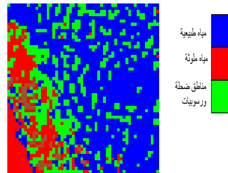
الشكل 7-: التصنيف الموجه (محطة مجاري السبيدية) للقمر Spot5
