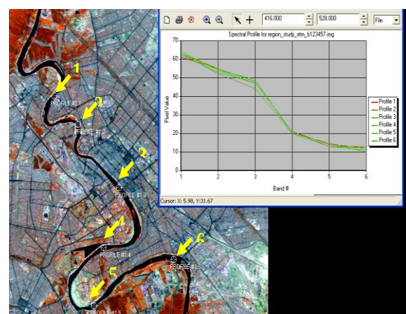
الشكل-2: التحليل الطيفي لصورة القمر الصناعي Land sat7 ETM+
