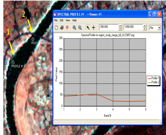
الشكل 4: التحليل الطيفي لموقع الجادرية ومحطة مجاري السديّة بعد اجراء عملية الدمج الحيزي لصورة القمر الصناعي Landsat7 ETM+
