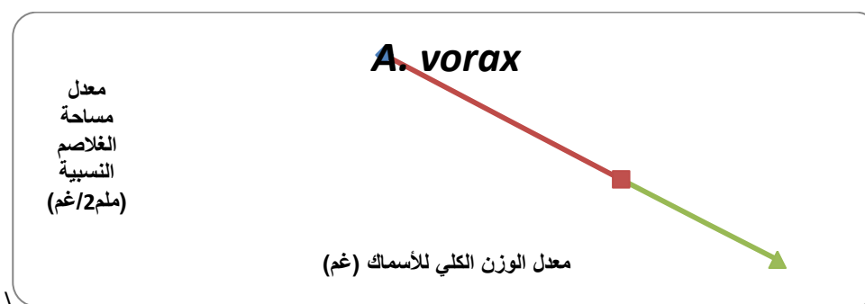
شكل (12) : يوضح العلاقة بين معدل الوزن الكلي للأسماك (ملم) ومعدل مساحة الغلاصم النسبية (ملم 2 /غم) في سمكة A. vorax .
