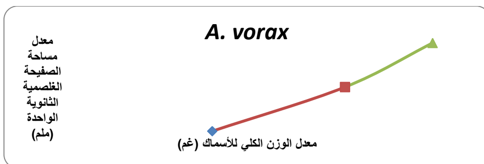
شكل (10) : يوضح العلاقة بين معدل الوزن الكلي للأسماك (ملم) ومعدل مساحة الصفيحة الثانوية الواحدة في سمكة A. vorax .
