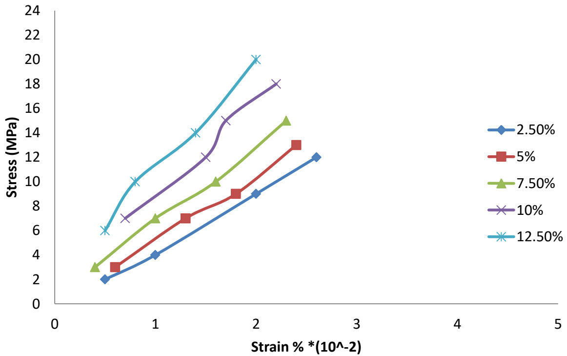
شكل (10) العلاقة بين الاجهاد-الانفعال لمترابك بوليمر - بنتونايت معالج بمادة PVA بوصفها دالة لكسور وزنية مختلفة عند درجة حرارة 500 °C
