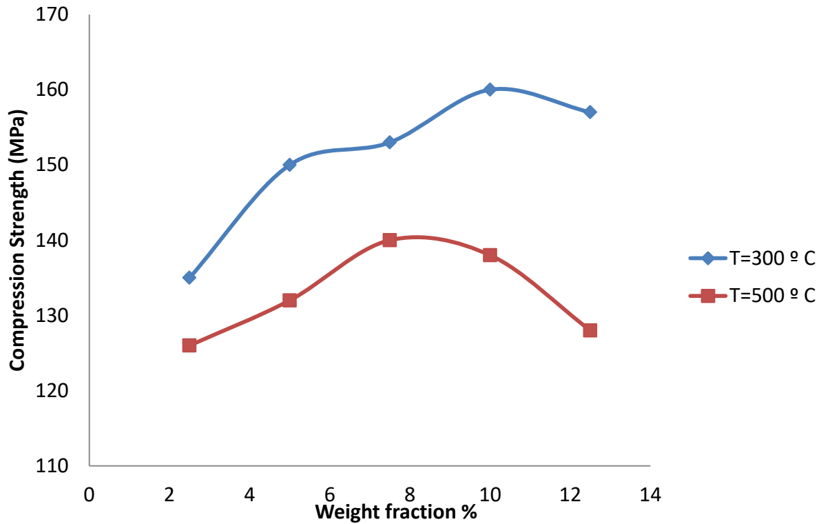
شكل (8) مقاومة الانضغاط لمركب بوليمر- بنتونايت معالج بمادة PVA بوصفها دالة لكسور وزنية مختلفة
