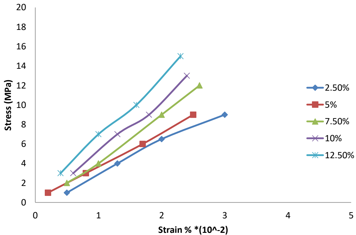
شكل (9) العلاقة بين الاجهاد-الانفعال لمركب بوليمر- بنتونايت معالج بمادة PVA بوصفها دالة لكسور وزنية مختلفة عند درجة حرارة 300 °C
