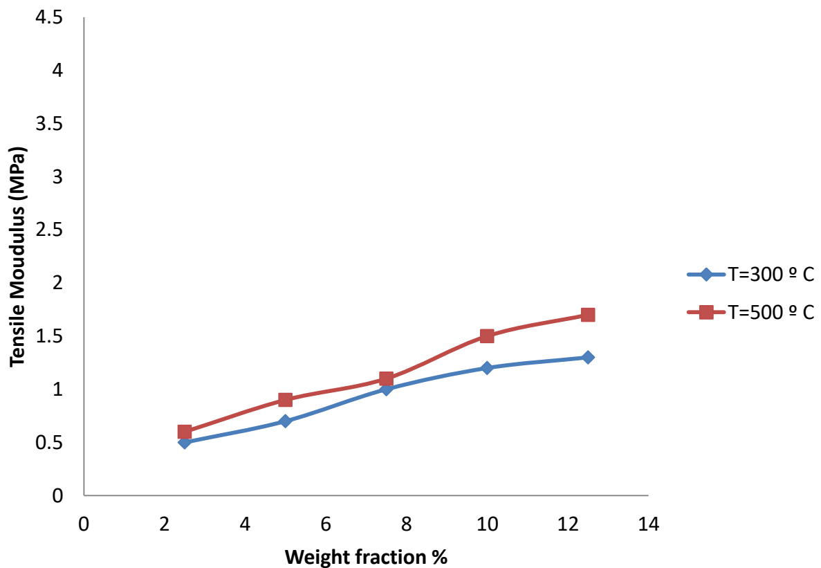
شكل (11) معامل مرونة الشد لمترابك بوليمر - بنتونايت معالج بمادة PVA بوصفها دالة لكسور وزنية مختلفة
