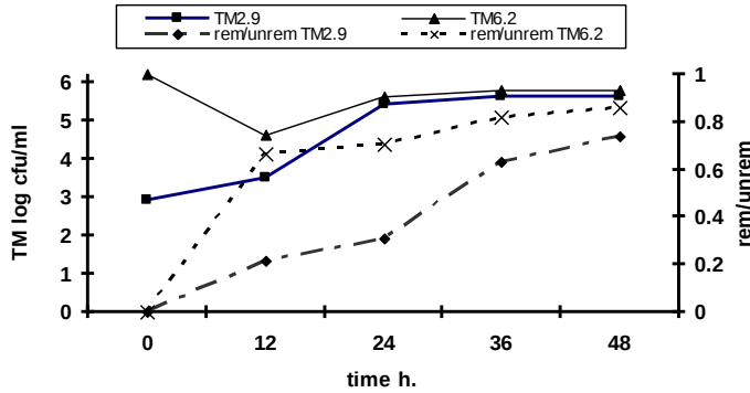
شكل-2: الكثافة الميكروبية ومعامل الإزالة لعنصر الكوبلت
