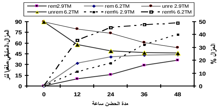
شكل-4: المزال والمتبقي ونسب المزال لعنصر الكادميوم خلال مدة الحضن
