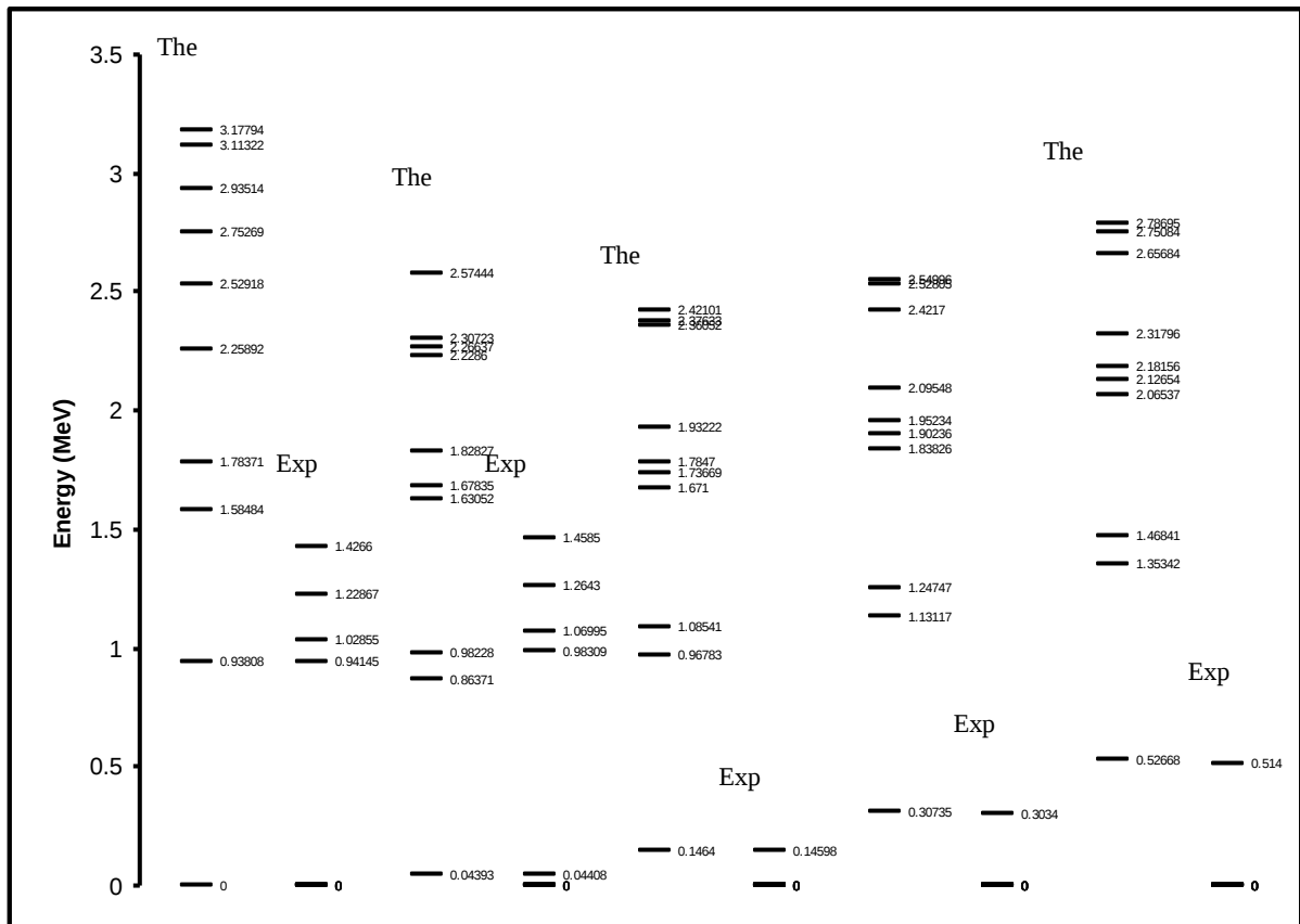
شكل (1) يمثل مستويات الطاقة العملية للنظير ^{238}\text{Pu} قورنت مع النتائج المستحصلة من البرنامج (IBM-1)
