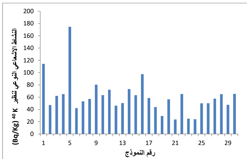
الشكل (3) الفعالية النوعية للبوتاسيوم ^{40}\text{K} في التربة السطحية cm (0-10)
