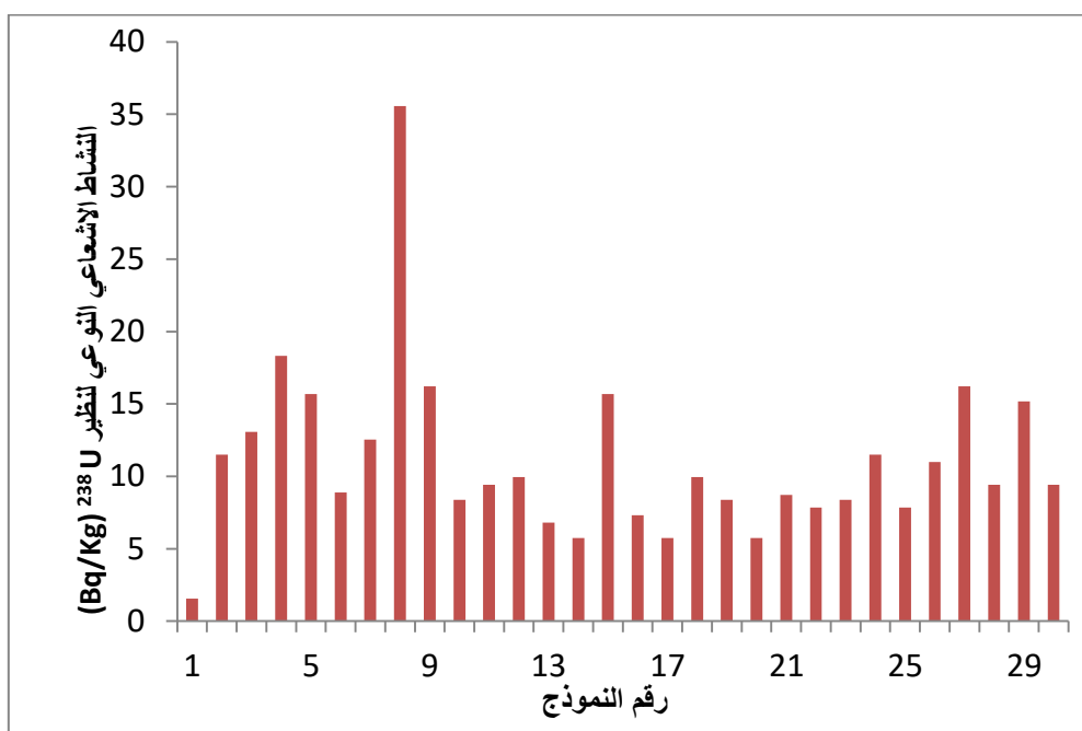
الشكل (6) الفعالية النوعية لليورانيوم ^{238}\text{U} لنماذج التربة بعمق cm(20-30)
