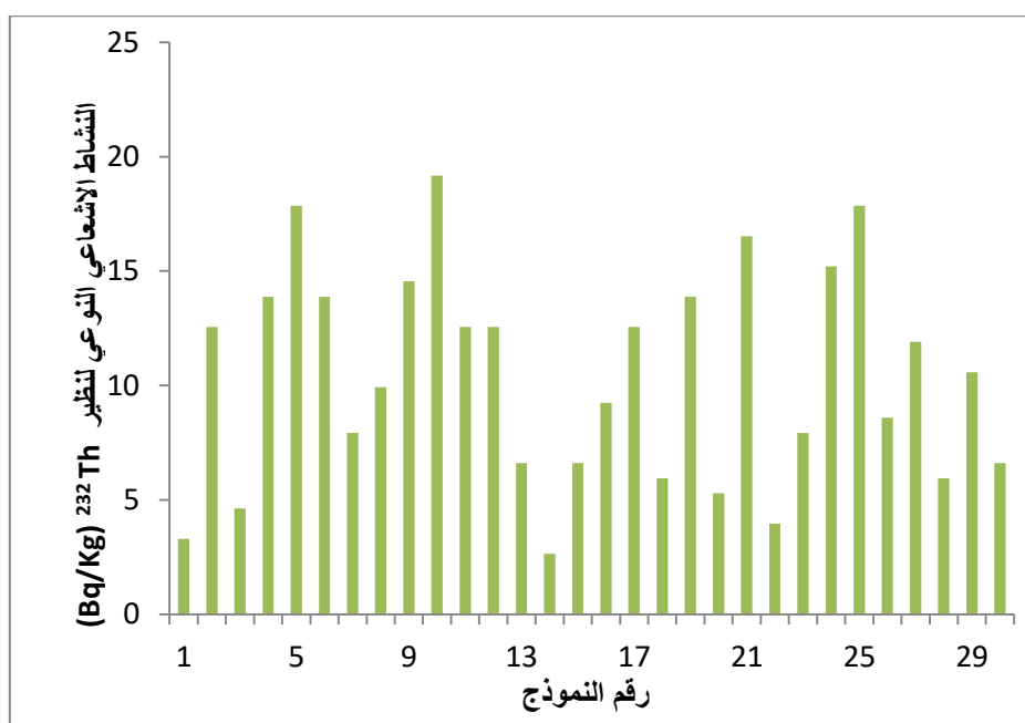
الشكل (8) الفعالية النوعية للثوريوم 232 Th لنماذج التربة بعمق (20-30)cm
