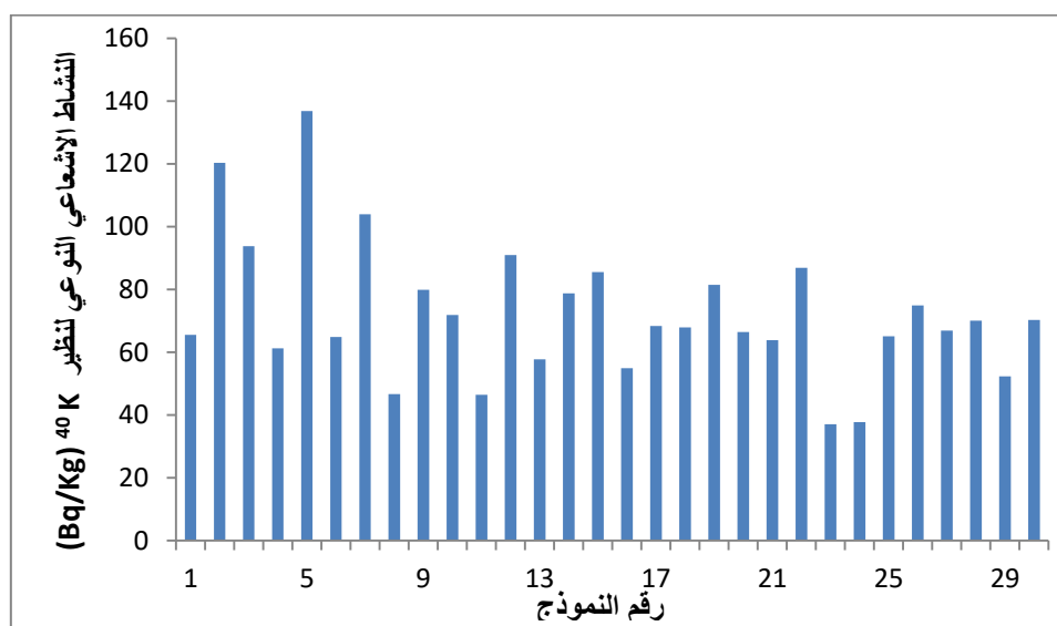
الشكل (4) الفعالية النوعية للبوتاسيوم ^{40}\text{K} لنماذج التربة بعمق cm (20-30)
