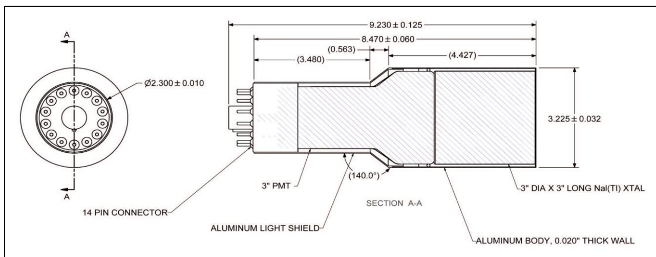
الشكل (2) يمثل تركيب الكاشف الوميضي
