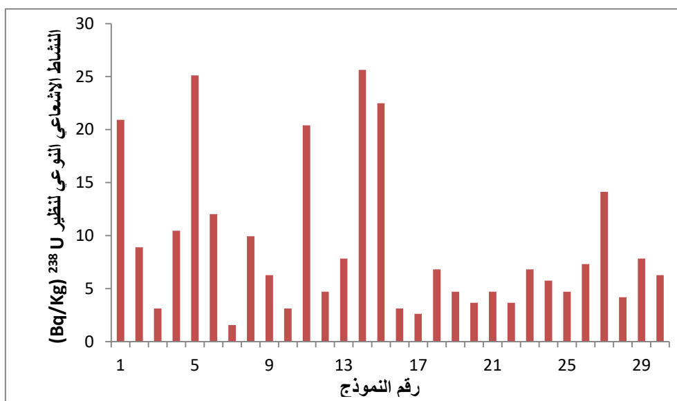
الشكل (5) الفعالية النوعية لليورانيوم ^{238}\text{U} في التربة السطحية cm(0-10)
