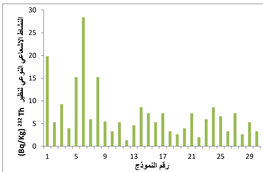
الشكل (7) الفعالية النوعية للثوريوم 232 Th في التربة السطحية (0-10)cm
