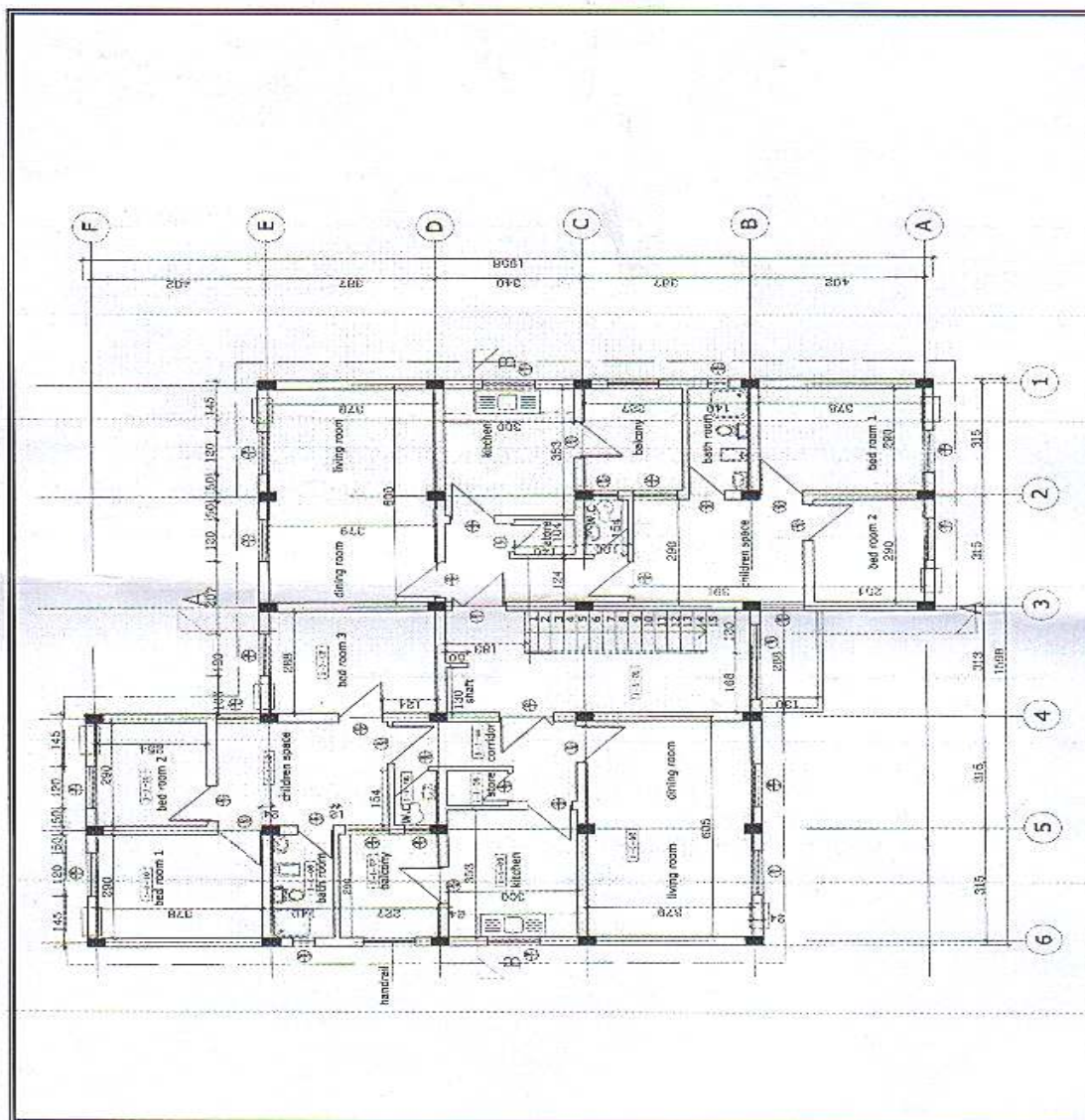
خارطة (1) لمجمع سبع ابار السكني في صدر القناة (الطابق الارضي) [ 15 ]
