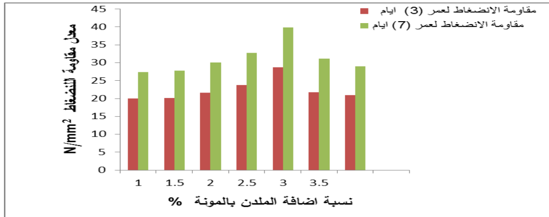
الشكل رقم (1) : العلاقة بين نسبة اضافة الملدن ومقاومة الانضغاط بمونة السمنت الممزوجة
