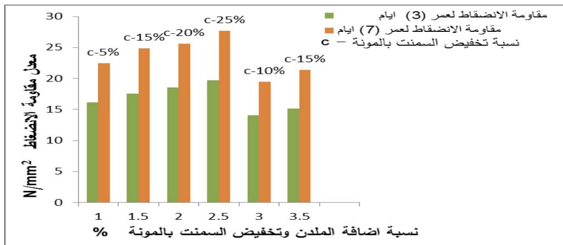
الشكل رقم (a-3) العلاقة بين نسبة الاضافة وتخفيض السمنت ومقاومة الانضغاط بالمونة الممزوجة
