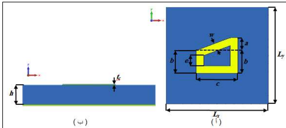
شكل رقم (1): (أ) منظر سطحي يوضح الأبعاد لخلية واحدة ، (ب) منظر جانبي.
