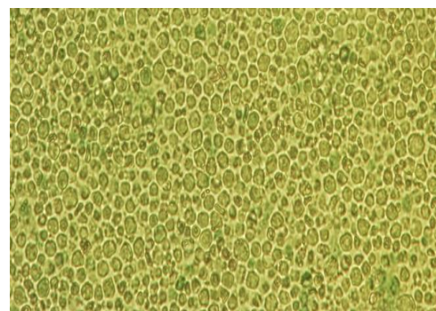
Control (0) μM
