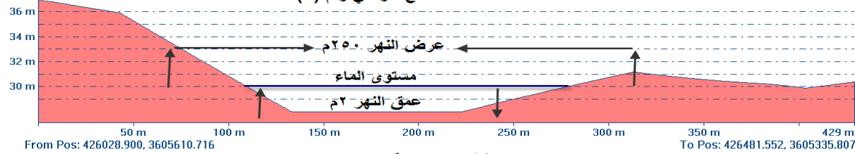
مقطع عرضي رقم (٤)
