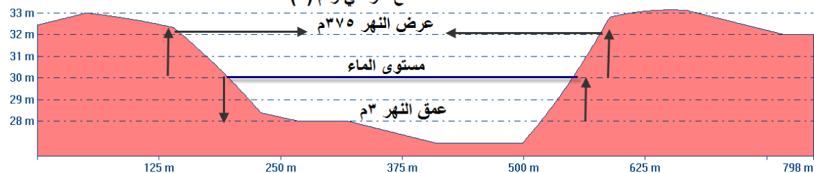
مقطع عرضي رقم (٦)
