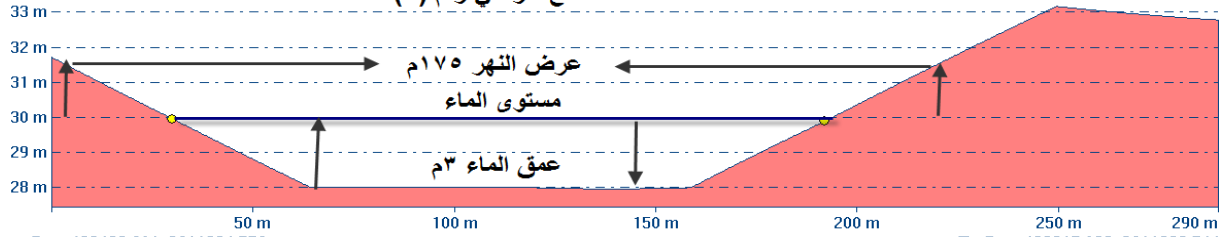
مقطع عرضي رقم (٢)
