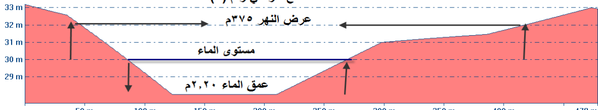
مقطع عرضي رقم (٦)
