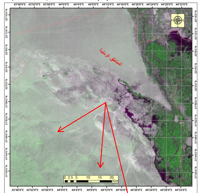
المرئية الفضائية (٢) التجمعات الرملية عام ٢٠١٧
