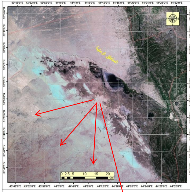
المرئية الفضائية (١) التجمعات الرملية عام ١٩٧٢
