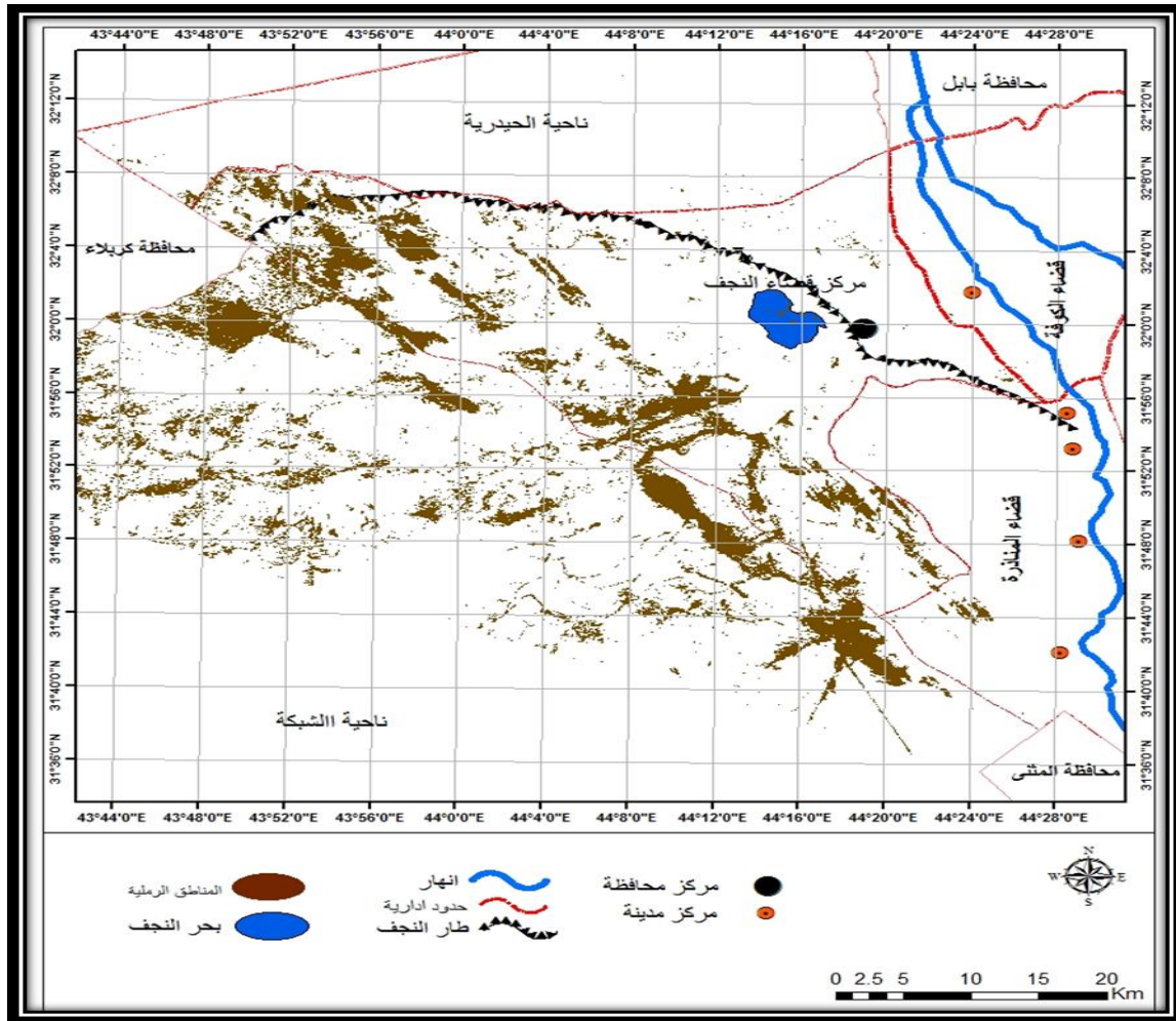
خريطة (١) التجمعات الرملية عام (١٩٧٢)
