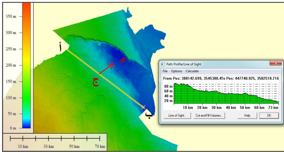
شكل (١) قطاع تضاريسي يبين انحدار السطح
