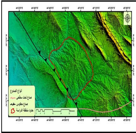
شكل (١) يوضح الصدع الانعكاسي (الانسري) ، شكل (٢) يوضح الصدوع التي تتأثر بها منطقة الدراسة تبعاً لحركته .
