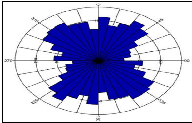
شكل ( ٩ ) يوضح اتجاه اعداد التراكيب الخطية لمنطقة الدراسة
