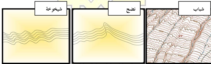
شكل ( ١١ ) يوضح المراحل العمرية لخطوط الكنتور تحليل شكل تعرج خطوط الكنتور Winding contour lines analysis :-
