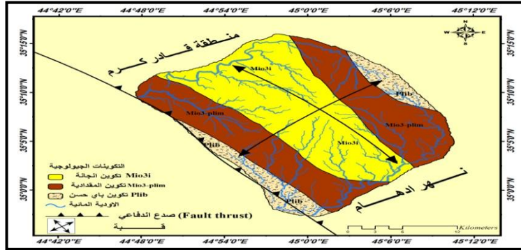
خريطة ( ٢ ) توضح جيولوجية منطقة الدراسة .
