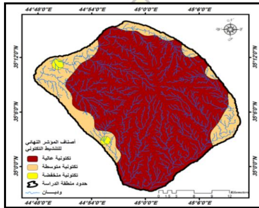
خريطة ( ١١ ) توضح التصنيف النهائي للمؤشرات الجيومورفولوجية لمنطقة الدراسة
