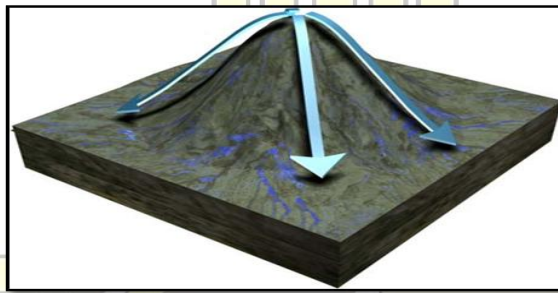
شكل ( ١٣ ) يوضح نمط التصريف الشعاعي (Radial).
