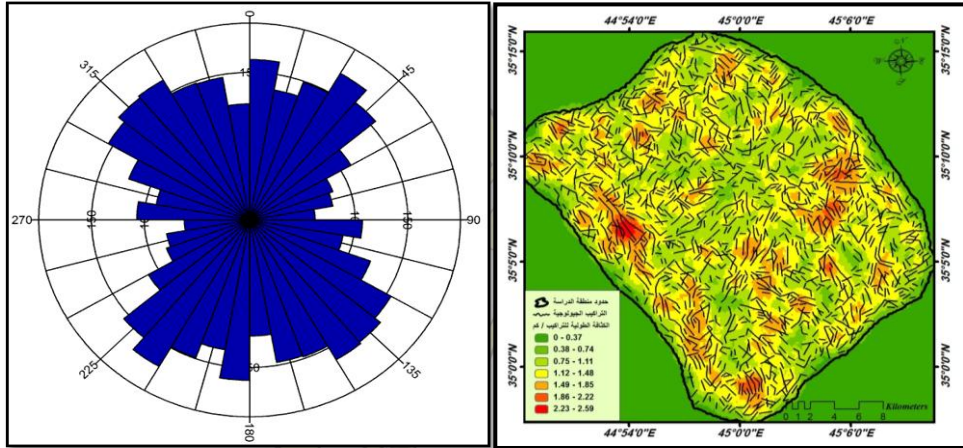
خريطة ( ٥ ) توضح كثافة واتجاه اطوال التراكيب الجيولوجية
