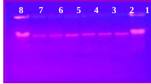
شكل ( 12 ) : الترحيل الكهربائي لنواتج تفاعل الانزيم المنقى جزئيا مع المادة الاساس (دنا الغدة الزعترية) بوجود احجام مختلفة من محلول اليوريا- 2 مركبتوايثانول على هلام الاكاروز بتركيز 0.8 % بفرق جهد 65 فولت ولمدة 1.5 ساعة.
