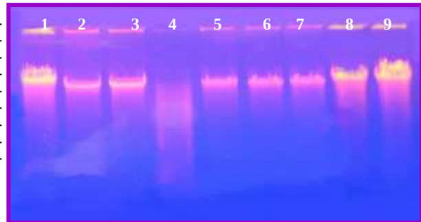
شكل (11): الترحيل الكهربائي لنواتج تفاعل الانزيم مع المادة الاساس (دنا الغدة الزعترية) بوجود تراكيز مختلفة من بعض المركبات الكيميائية على هلام الاكاروز بتركيز 0.8 % بفرق جهد 65 فولت ولمدة 1.5 ساعة.
