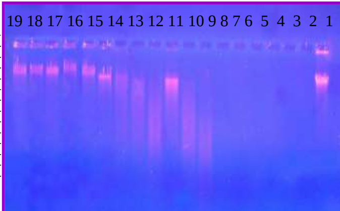
شكل (10): الترحيل الكهربائي لنواتج تفاعل الانزيم مع المادة الاساس (دنا الغدة الزعترية) بوجود تراكيز مختلفة لمحاليل بعض الايونات على هلام الاكاروز بتركيز 0.8 % بفرق جهد 65 فولت و لمدة 1.5 ساعة .
