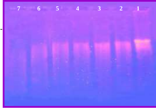
شكل ( 5 ) : الترحيل الكهربائي لنواتج تفاعل الانزيم المنقى جزئياً مع المادة الاساس(دنا الغدة الزعترية) باوقات حضانة مختلفة على هلام الاكاروز بتركيز 0.8 % بفرق جهد 65 فولت ولمدة 1.5 ساعة
