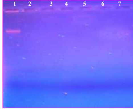
شكل ( 2 ) : الترحيل الكهربائي لنواتج تفاعل الانزيم مع المادة الاساس (دنا الغدة الزعترية) لتحديد التركيز الامثل للانزيم الخام على هلام الاكاروز بتركيز 0.8 % بفرق جهد 65 فولت ولمدة 1.5 ساعة .
