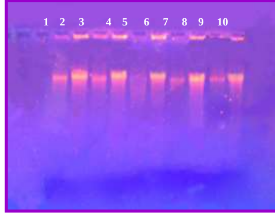
شكل (7): تفاعل الانزيم مع المادة الاساس (دنا الغدة الزعترية) لتحديد الرقم الهيدروجيني الامثل لفعالية الانزيم على هلام الاكاروز بتركيز 0.8 % بفرق جهد 65 فولت ولمدة 1.5 ساعة.
