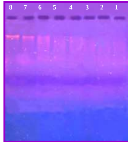
شكل ( 3 ) : الترحيل الكهربائي لنواتج تفاعل الانزيم مع المادة الاساس (دنا الغدة الزعترية) باوقات حضن مختلفة على هلام الاكاروز بتركيز 0.8 % بفرق جهد 65 فولت و لمدة 1.5 ساعة .
