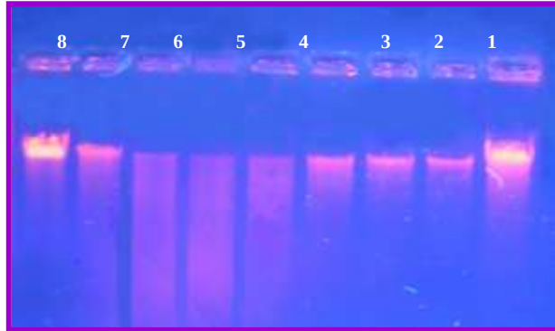
شكل (9): تفاعل الانزيم مع المادة الاساس (دنا الغدة الزعترية) لتعيين الدرجة الحرارية المثلى لفعالية الانزيم المنقى جزئياً على هلام الاكاروز بتركيز 0.8 % بفرق جهد 65 فولت ولمدة 1.5 ساعة .
