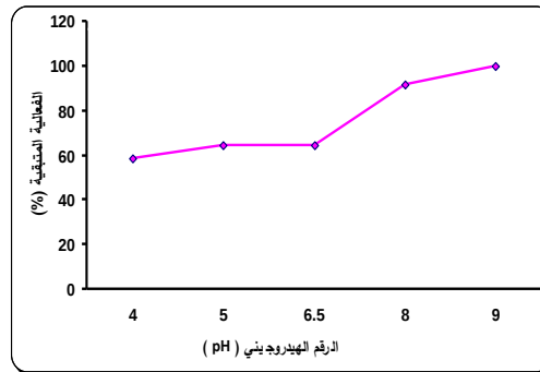
شكل (8): تأثير قيم مختلفة من الرقم الهيدروجيني (4 - 9) في ثباتية الانزيم DNase I البكترياسي
