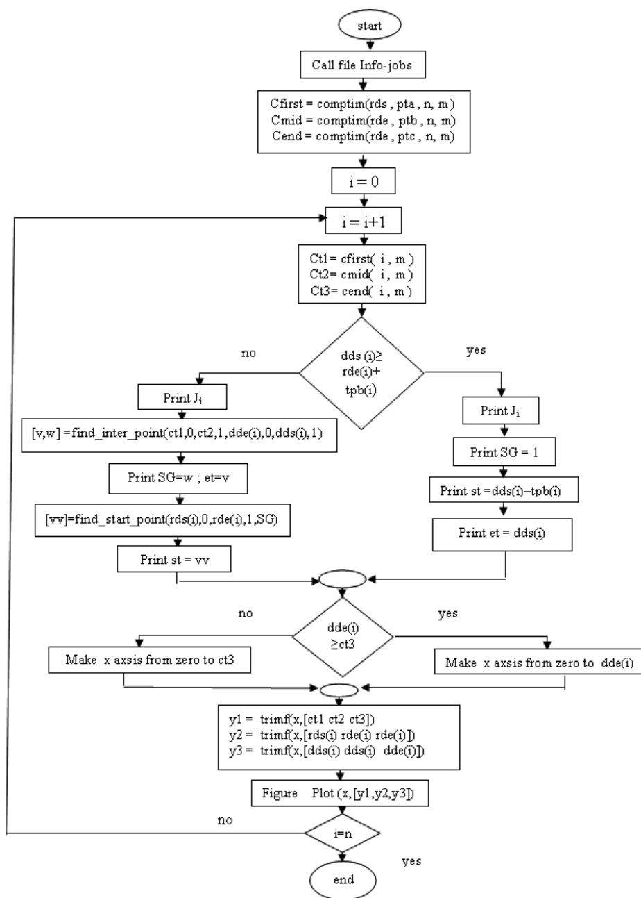
الشكل (6): المخطط الانسيابي للخوارزمية المصممة
