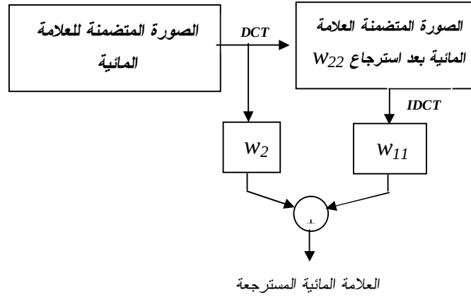
الشكل (5): خوارزمية الاسترجاع المجهن
