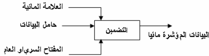
الشكل(1): المخطط العام للتأشير المائي الرقمي
