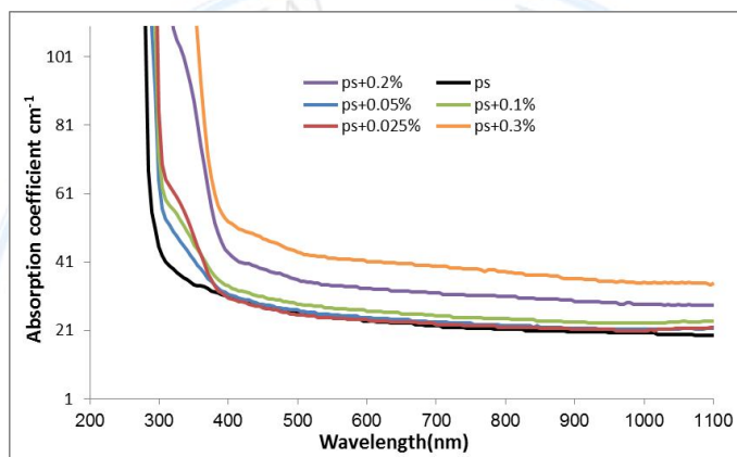
الشكل (2) يوضح معامل الامتصاص كدالة للطول الموجي لأغشية (ps) النقية والمشوبة
