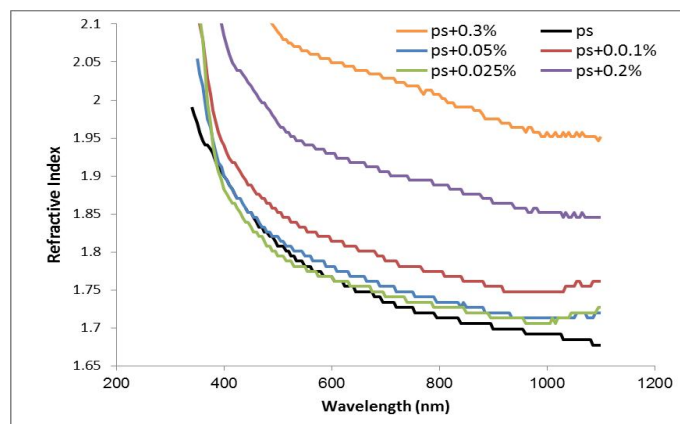
الشكل (4) يوضح معامل الانكسار كدالة للطول الموجي لأغشية (ps) النقية والمشوبة
