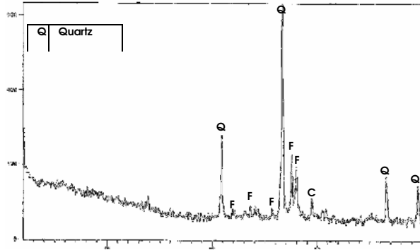
شكل (6) مخطط (X.R.D) للحبيبات (0.125-0.25mm) في مقطع الزبير (Z3).
