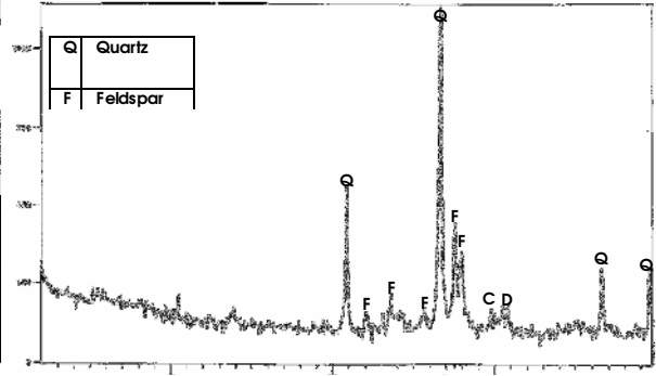
شكل (5) مخطط (X.R.D) للحبيبات (0.125-0.25mm) في مقطع سفوان (S3).
