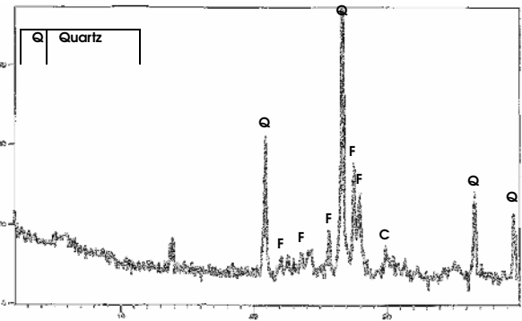
شكل (7) مخطط (X.R.D) للحبيبات (0.25-0.5mm) في مقطع سفوان (S3).
