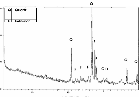
شكل (11) مخطط (X.R.D) للحبيبات (1-2mm) في مقطع سفوان (S3).
