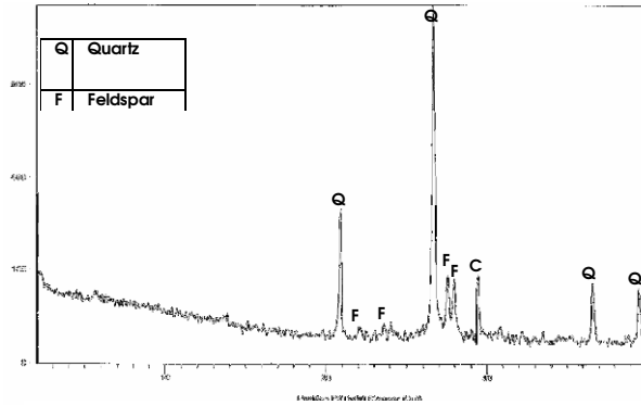
شكل (8) مخطط (X.R.D) للحبيبات (0.25-0.5mm) في مقطع لزبير (Z3).
