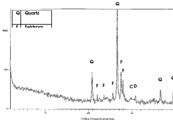
شكل (12) مخطط (X.R.D) للحبيبات (1-2mm) في مقطع الزبير (Z3).
