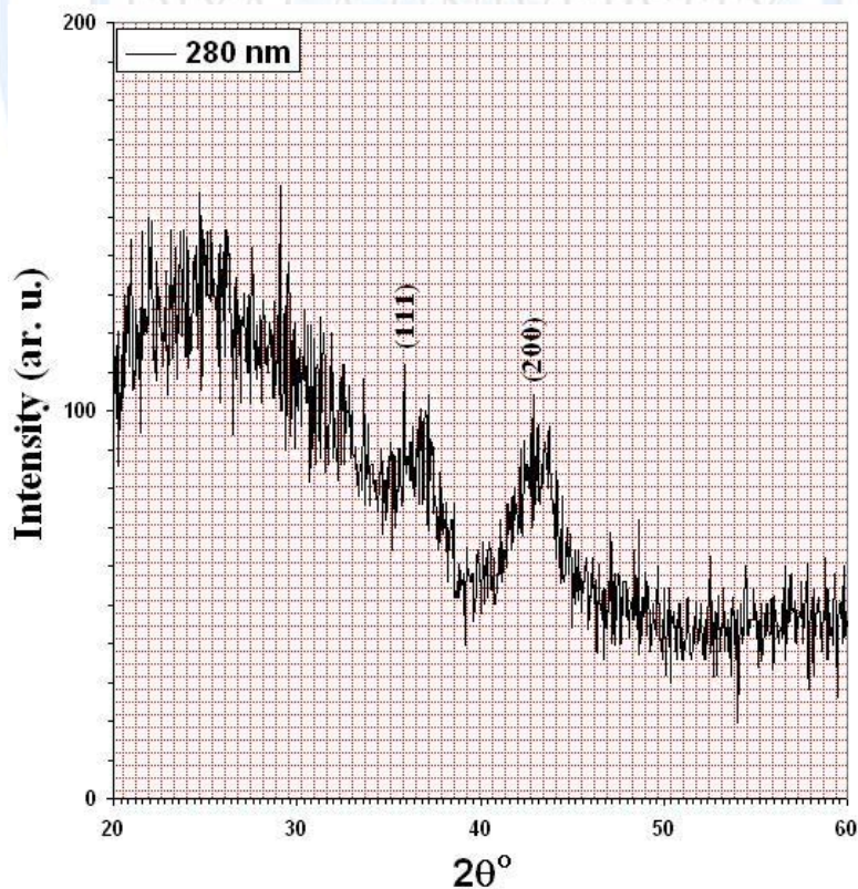
الشكل (4) مخطط حيود الأشعة السينية لغشاء NiO بسمك (280nm).
