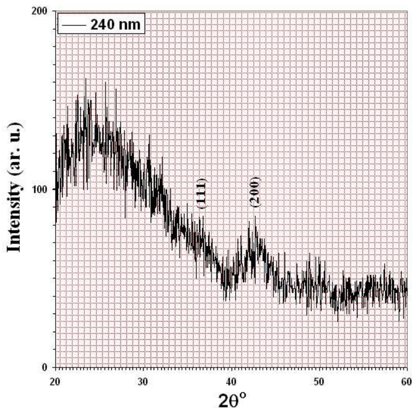
الشكل (3) مخطط حيود الأشعة السينية لغشاء NiO بسمك (240 nm).
