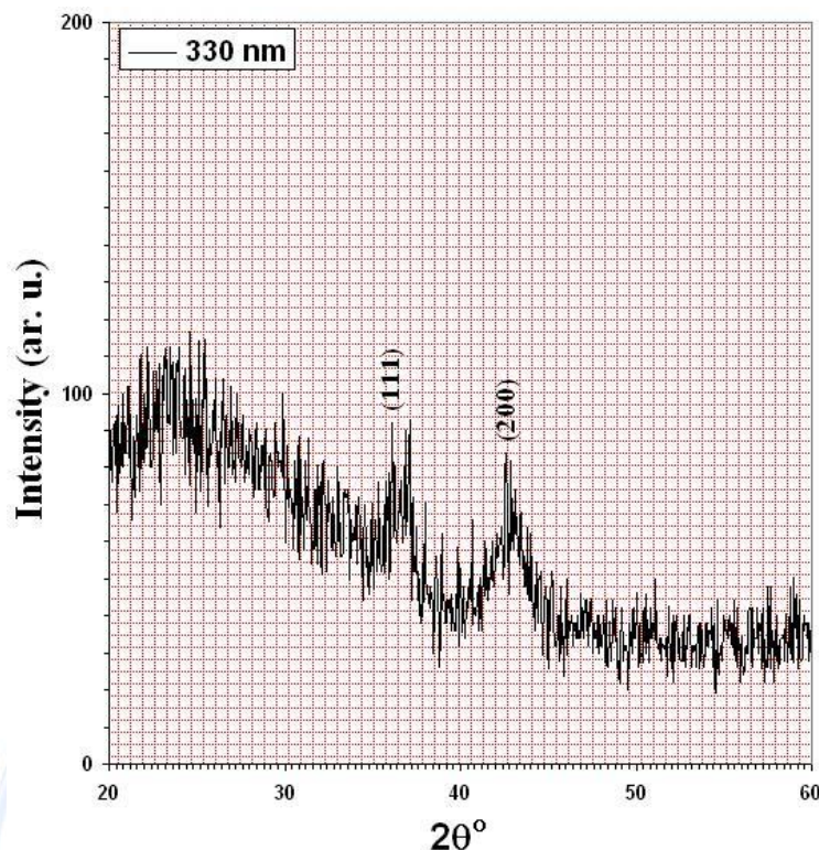
الشكل (5) مخطط حيود الأشعة السينية لأغشاء NiO بسمك (330 nm).
