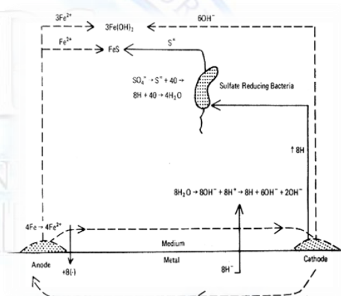
شكل (١) آلية التآكل الحيوي لحديد التسليح بفعل البكتريا المختزلة للكبريت (Coetser and Cloete, 2005)
