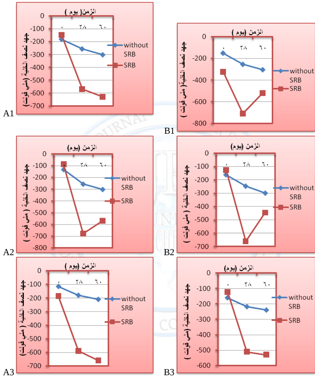
شكل (5) مقارنة سرعة التآكل بين عينات الزرع وعينات السيطرة للنماذج (A1,A2,A3) للخلطة الاعتيادية ومقارنة سرعة التآكل للنماذج (B1,B2,B3) مع عينات السيطرة للخلطة عالية المقاومة
