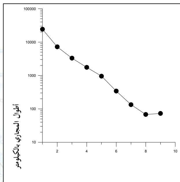
أ- رتب نهريه مع اطوال المجاري الرتبة النهرية
