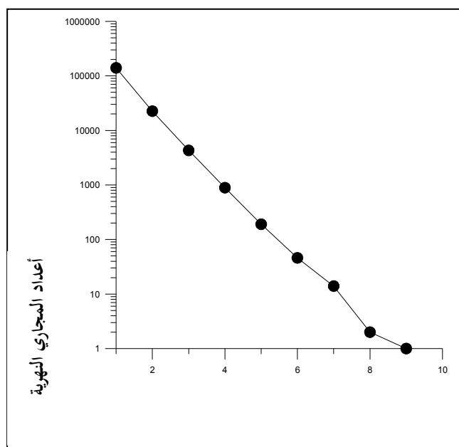
ب- رتب نهريه مع اعداد المجاري الرتبة النهرية
