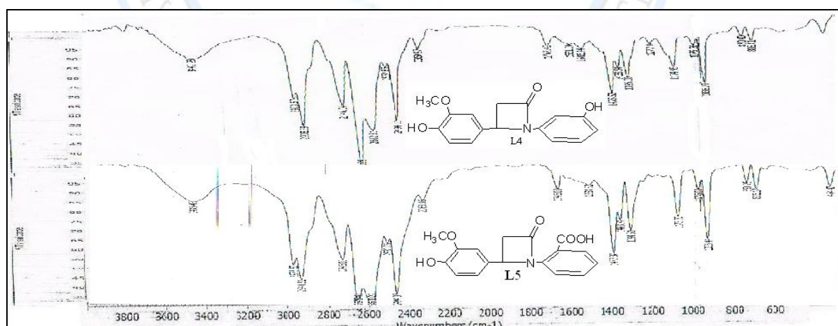
شكل (٤) أطياف FTIR لمركبات ألبيتا لاكتام أحادية الحلقة
