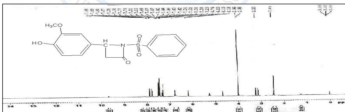
الشكل (٥) طيف ^1\text{H} NMR لمركبات لبيتا لاكتام
