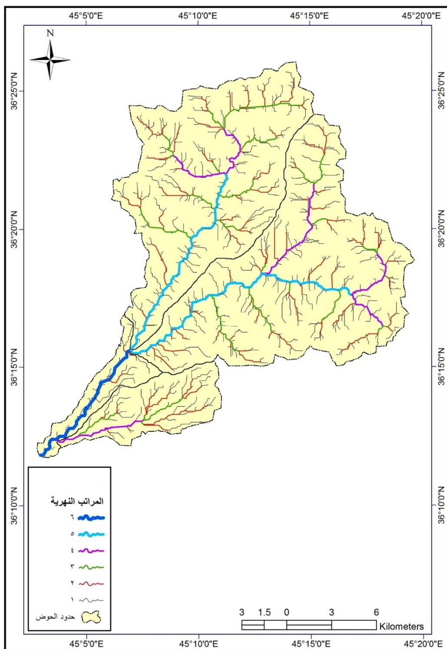
خريطة (5) المراتب النهرية لحوض ذراوة
