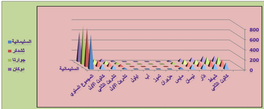
شكل بياني (٢) المعدلات الشهرية والمجموع السنوي للأمطار (ملم) في محطات منطقة الدراسة
