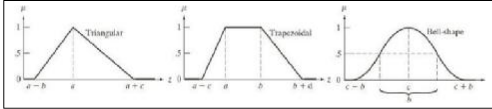
الشكل (٣) يوضح أشكال بعض دوال العضوية
