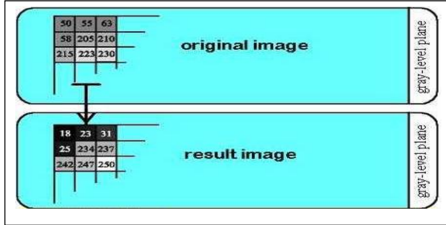
الشكل (5) يوضح عملية تحسين التباين في الصور باستخدام المنطق المضبيب
