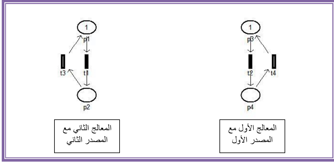
مخطط (2) يمثل معالجات مع مصدرين باستخدام Petri Net
