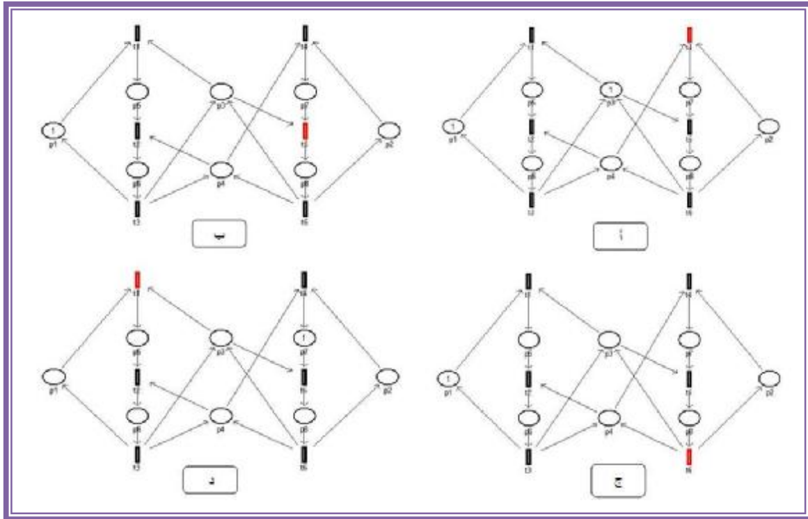
مخطط (4) تنفيذ سلسلة من عمليات الـ firing
