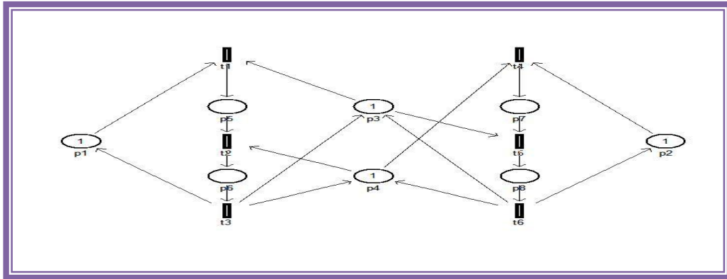
مخطط (3) عملية مشاركة المصدرين لكلا المعالجات
