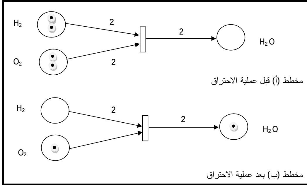
مخطط (1) توضيح معادلة الماء الكيميائية باستخدام Petri Net
