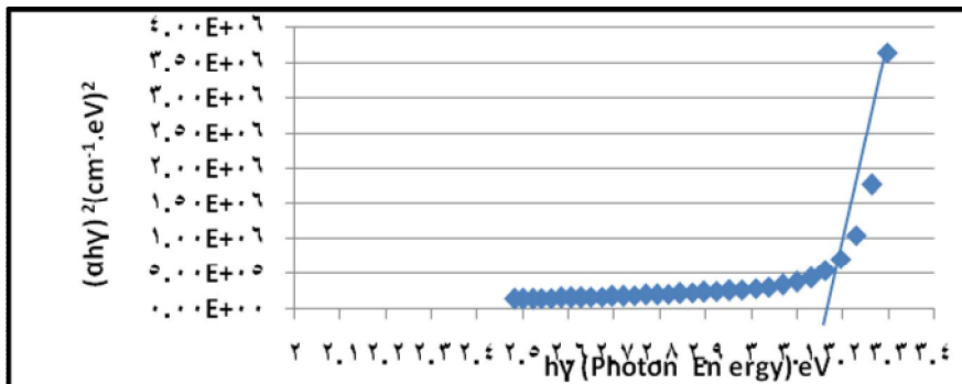
شكل (4-a): فجوة الطاقة للغشاء ZnO (t=300Å) بعد ( 90 min ) من التشعيع ، E_g = (3.17) \text{ eV} .
