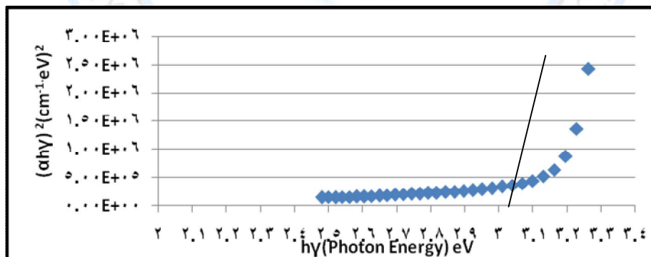
شكل (5-a): فجوة الطاقة للغشاء ZnO (t=300Å) بعد ( 1410 min ) من التشعيع ، E_g = (3.14) \text{ eV} .
