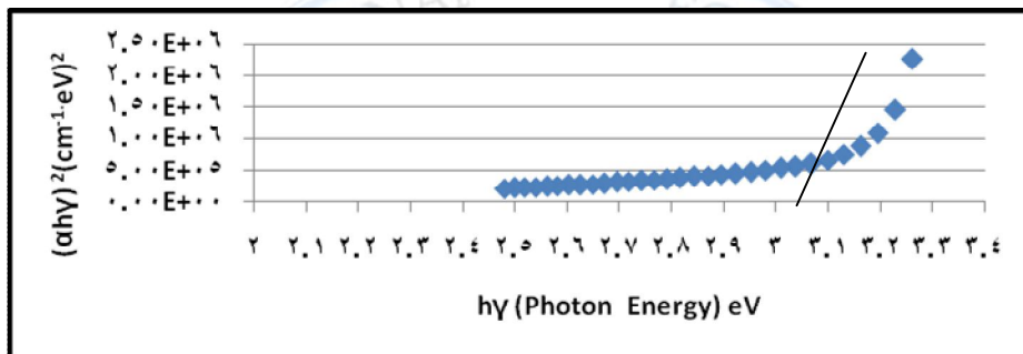
شكل (4-b): فجوة الطاقة للغشاء ZnO (t=1500Å) بعد ( 90 min ) من التشعيع ، E_g = (3.15) \text{ eV} .
